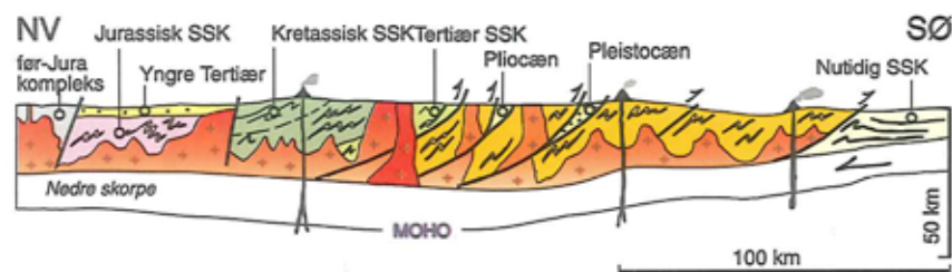
Figur 6. Skematisk profil gennem den øvre litosfære i den japanske øbue (Honshu). Jordskorpen opbygges af sammenskudte jurassiske til kvartære 'skrab-sammen-kiler' (SSK), gennemsat af opstegne granitiske magma-bjergarter. Bjergarternes alder aftager generelt i sydøstlig retning - mod subduktions- zonen. I den nedre skorpe optræder der bl.a. gabbro og amfibolit.
