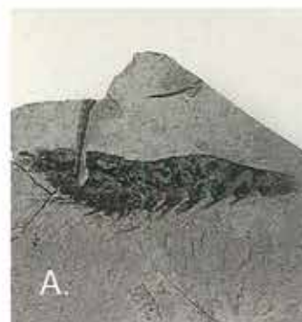
A) Den største og flotteste reje (3.5 cm lang) fra 'skiferen' tilhørende gruppen af penaeider. Foto: S.L.Jacobsen. B) Pyrit-imprægneret unge af en ny art beslægtet med glansfisk. Flot præpareret af H. Madsen, så de lange stråler i bugfinnerne ses. Foto: O.B.Berthelsen.
