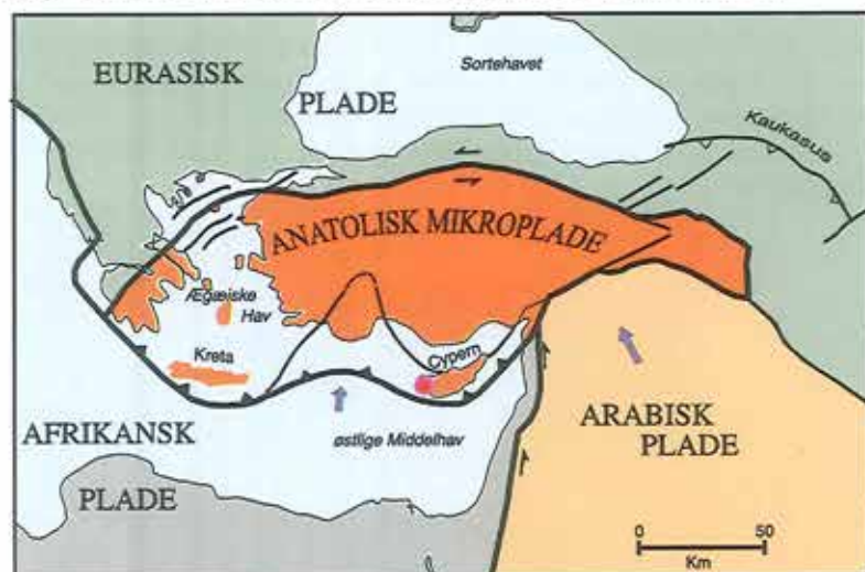
Fig. 2. De pladetektoniske forhold omkring Cypern og det østlige Middelhav. Den afrikanske plade subduceres under den anatolske, mens den hurtigere arabiske plade får den anatolske til at rotere mod uret. Derved strækkes, normal-forkastes og fortyndes jordskorpen under det nordlige Ægæiske Øhav. Den nord-anatolske forkastning danner nordgrænsen for plade-rotationen.
