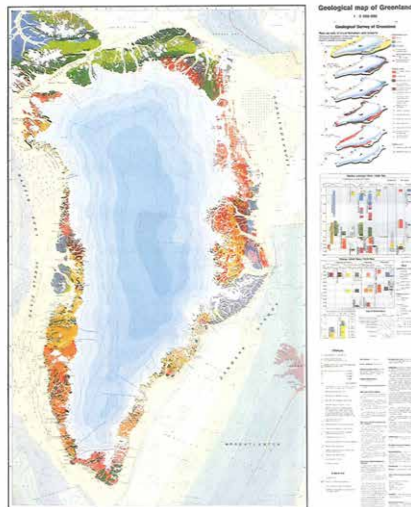
Det nye geologiske kort over Grønland.
