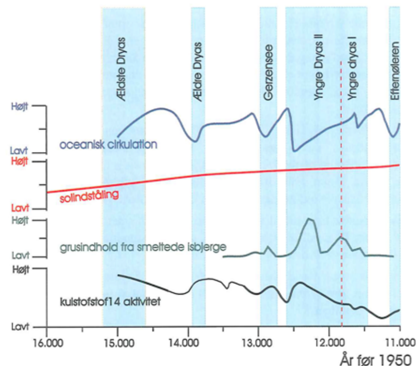
Figur 11. Klimaudviklingen fra Ældste Dryas til 'Efternøleren' illustreret ved data fra ENAM 93-21 borekernen fra 1000 meters dybde ud for Færøerne. Solindstrålingen er steget jævnt siden 20.000 år før nutid. Indholdet af grus fra smeltede isbjerge varierer, og ^{14}\text{C} -aktiviteten i atmosfæren følger næsten samme trend, men aftager og stiger modsat den oceaniske cirkulation. Nederst er vist de kolde perioders længde og navne. Yngre Dryas omfattede en første meget kold del (I) og en senere lidt varmere del (II).
