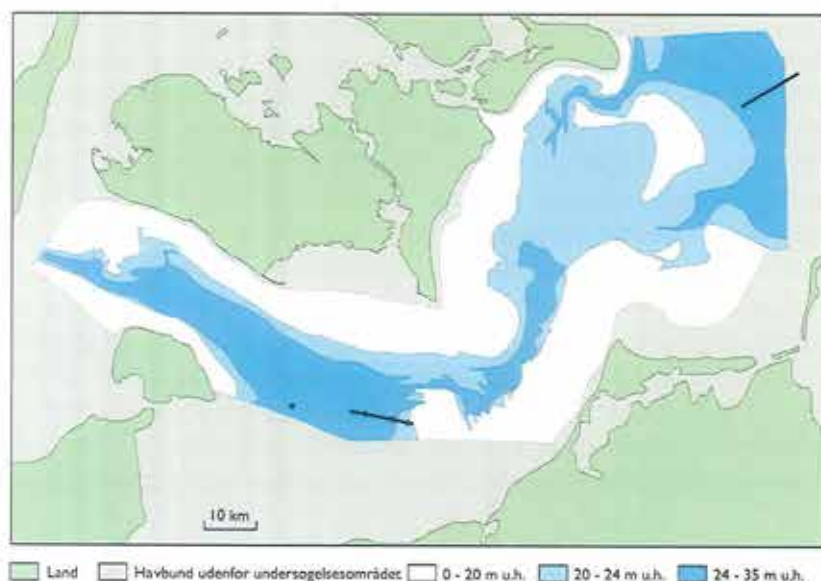
Figur 4. Den senglaciale overflademorfologi, som den tager sig ud i dag. De postglaciale sedimenter er 'fjernet'. Der har været to forbindelser til Østersøen øst for Darss Tærsklen, men den nordligste er den dybeste og har spillet den største rolle. Beliggenheden af de seismiske profiler og kerner på figur 5 og 6 er også vist.
