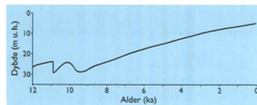
Figur 8. Model for udviklingen af de relative vandspejlsændringer i Mecklenburg Bugt vest for Darss Tærsklen. Det relative vandspejl er steget godt 25 meter siden tidlig Holocæn, men da verdenshavens vandspejl er steget ca. 50 meter inden for samme tidsrum, må den isostatiske hævn i området andrage ca. 25 meter. Bemærk, at der er registreret et fald i vandstand efter Ancylus Søens maksimum på højst 5 meter.
