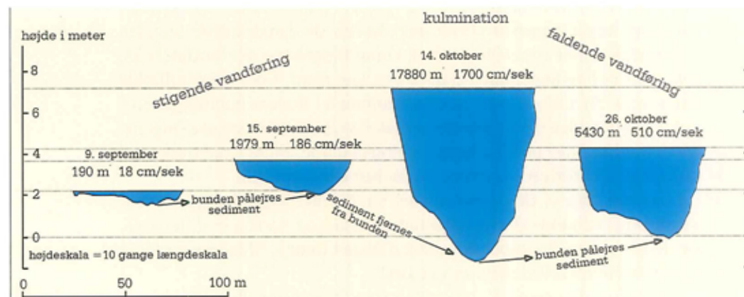
Variationer i en strømkanaals form i løbet af en periode med faser af lav vandstand -stigning af vandet - kulmination - sænkning af vandet. Strømningshastigheden (centimeter per sekund) og den per sekund transporterede vandmasse i kubikmeter fremgår ligeledes af figuren.
