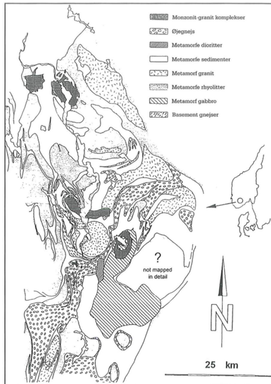
Forenklet kort over Setesdalområdet (delvis baseret på Sigmond (1975) og Falkum (1982)).
