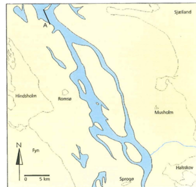
Storebælt for ca. 9.600 år f.Kr., hvor bæltet var bevokset med tundra, og store langstrakte søer fyldte det centrale dalsystem. Se anmeldelse i VARV 1998, 4.
