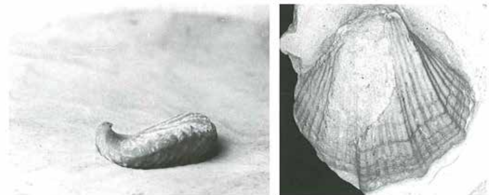
Figur 35: tv.) Halvkugleformet armsfod (Trigonosemus pulchellus) anbragt som den har ligget på kridtbunden. th.) Muslingen Neitheia sexcostata stærkt hvælvede underskal, ca 2,5 cm
