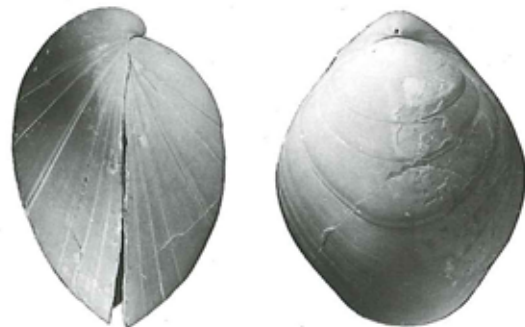
Figur 36. Kugleformet armfod ('tumling'), Carneithyris subcardinalis , naturlig størrelse. Til venstre i livsstilling på kridtbunden.
