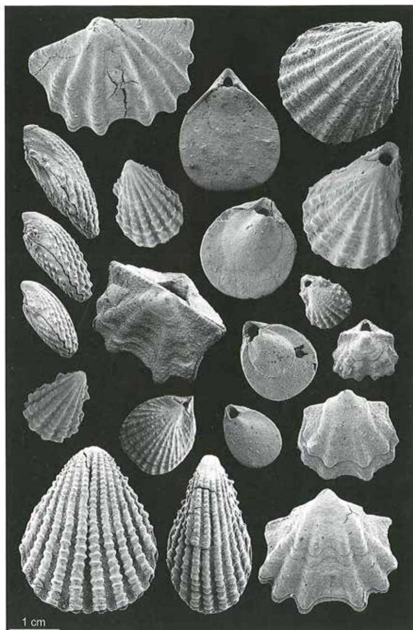
Figur 50. Et udvalg af skrivekridtets mange små armfodder. Alle viste eksemplarer har siddet fasthæftet ved hjælp af en stilk, som stak ud gennem stilkåbningen i den ene skal.
