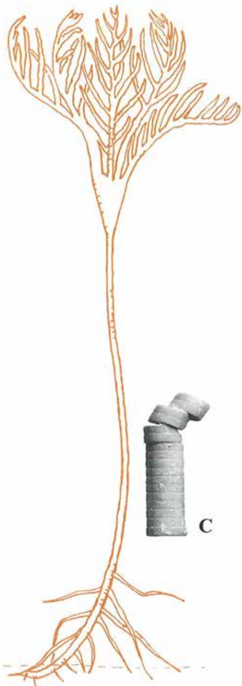
Figur 39. Søilje. Plader fra forskellige søiljer fra henholdsvis krone (A) og stilk (B & C), samt skitse af søilje, der lever rodfæstet i en blød bund. Stilkleddene, der kan være fra runde til stjerneformede, er ca. 1 centimeter i diameter. Armleddene (øverst) er noget mindre.
