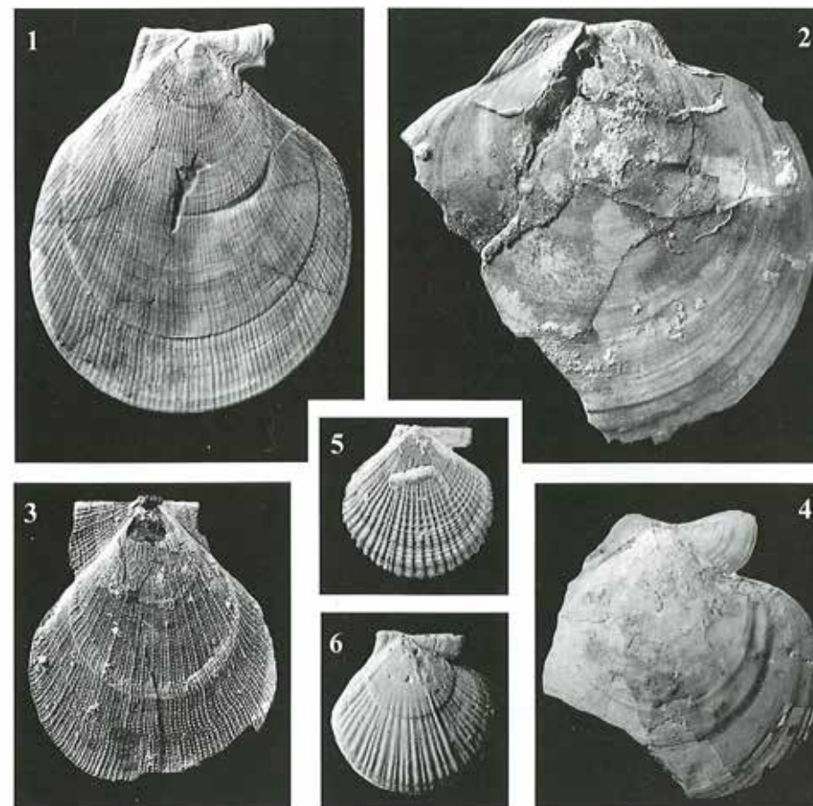
Figur 43. Kammuslinger. Alle har kunnet svømme, nogle bedre end andre.
