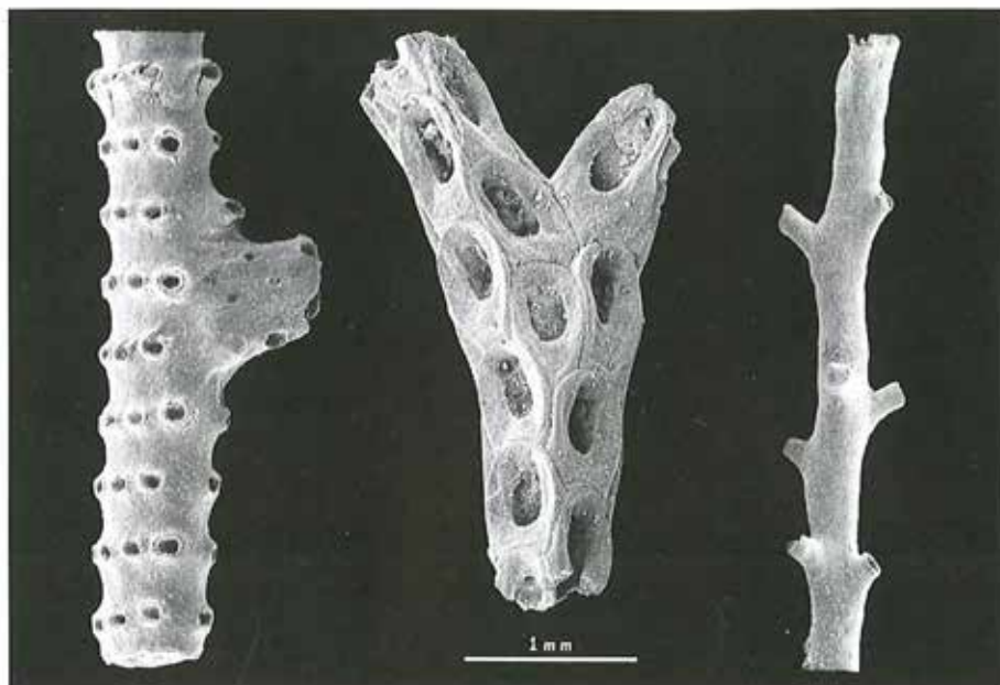
Figur 42. Mosdyrkolonier. Eksempler på tre af de grentyper, som forekommer i kridtet. Nederfor ses en nulevende grenet koloni.
