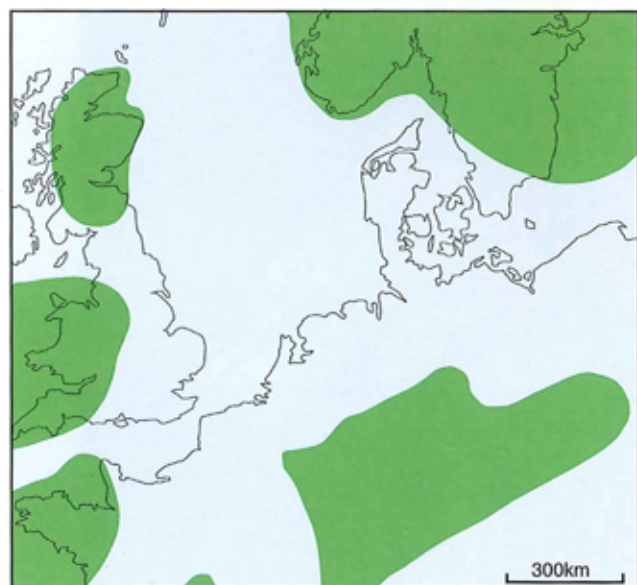
Figur 2. Nordeuropa i Kridttidens sidste del for ca. 70 millioner år siden. De blå områder er hav, de grønne land.
