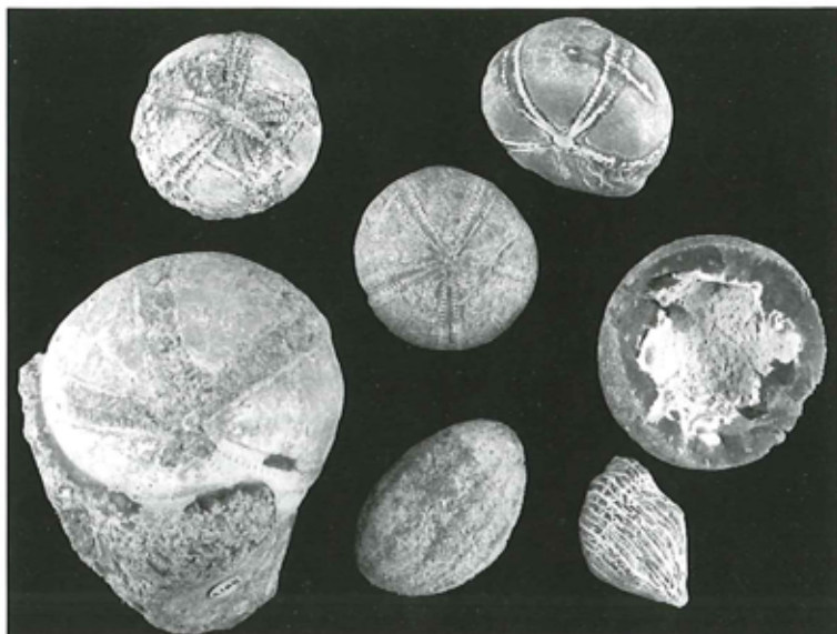
Figur 4. Forskellige fossiler bevaret i flint. Et stort søpindsvin, 3 små, yderst til højre en halv raslesten, derunder en koral og nederst i midten et stykke af en svamp ( Aulaxinia ).
