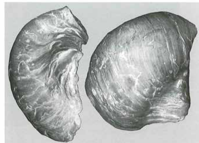
Figur 31. Underskallen af østersen Pycnodonte vesiculare . Skallens længde er ca. 10 centimeter
