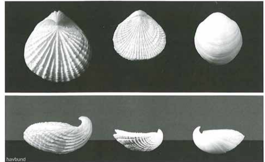
Figur 34 Tre halvkugleformede armsfodder: Trigonosemus pulchellus, Terebratulina gracilis og Magas chitoniformis. Alle tre har de levet med den hvælvede skal nede i det bløde kridtslam. Det største af dyrene er ca. 8 millimeter langt.
