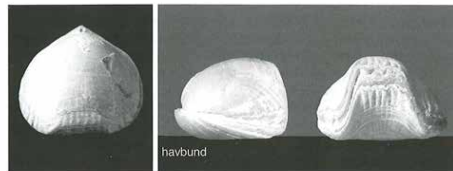
Figur 27. Armfoden Cretirhynchia retracta . Dyret lå på sin flade skal. På billedet til venstre ses stilkhullet, som hos det voksne individ er lukket indefra. Til højre ses den kraftigt ophvælvende skalrand, som sikrer adskillelse af ind- og udåndingsvandet. Randens fine takker fungerede som filter mod indtrængende partikler.
