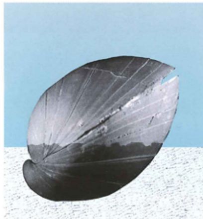
Figur 36. Kugleformet armfod ('tumling'), Carneithyris subcardinalis , naturlig størrelse. Til venstre i livsstilling på kridtbunden.
