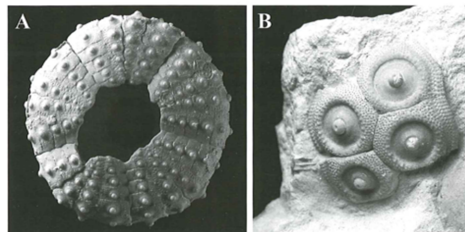
Figur 23 A. Skal af regulært søpindsvin af slægten Phymosoma , set fra undersiden (diameter ca. 5 centimeter). 23B. Plader fra skal af regulært søpindsvin af slægten Cidaris . De runde knuder i midten af de cirkulære felter (sopatter!) var hæfte for de kraftige og meget bevægelige pigge, som karakteriserer denne gruppe søpindsvin.
