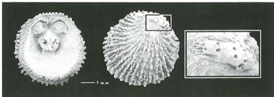
Figur 56. Isocrania costata , en stilkløs armfod der begynder tilværelsen som cementeret på et hårdt substrat, her et stykke af en mosdyrkoloni. Efterhånden som armfoden vokser, kommer den til at ligge frit på bunden.
