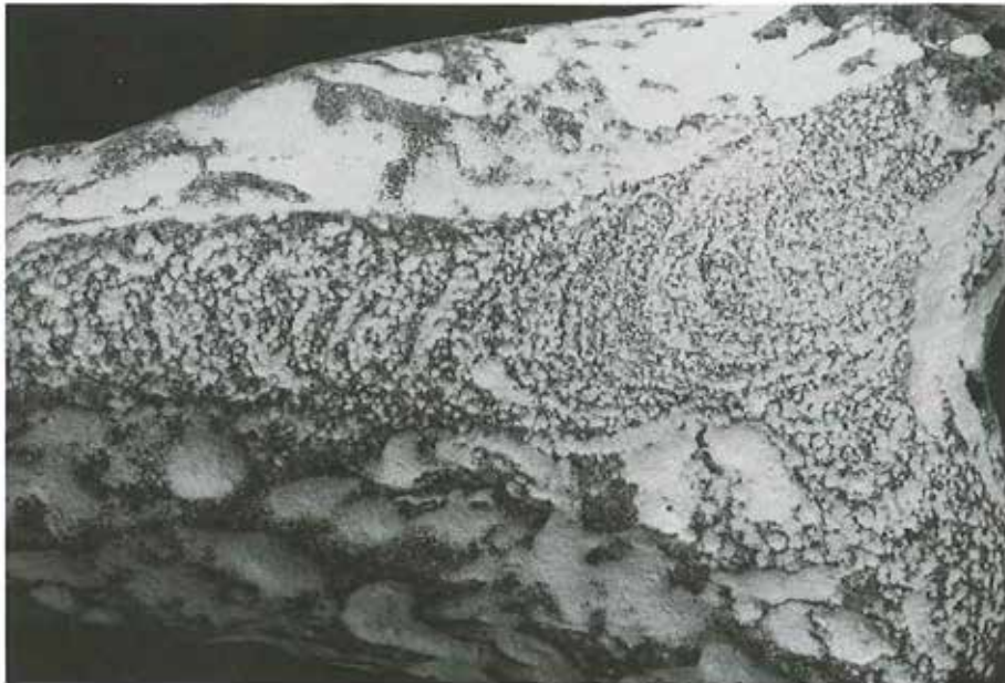
Figur 18. Gravesporet Taenidium (ca. 1 o centimeter i diameter) bevaret på overfladen af en flintknold. De halvmåneformede figurer er de portioner af sediment, som dyret har pakket bag sig, efterhånden som det gravede sig gennem sedimentet. Selve flintknolden er udfyldningen af en Thalassinoides gang. De runde hvide pletter under Taenidium sporet kan være markeringer efter Chondrites (se figur 17).
