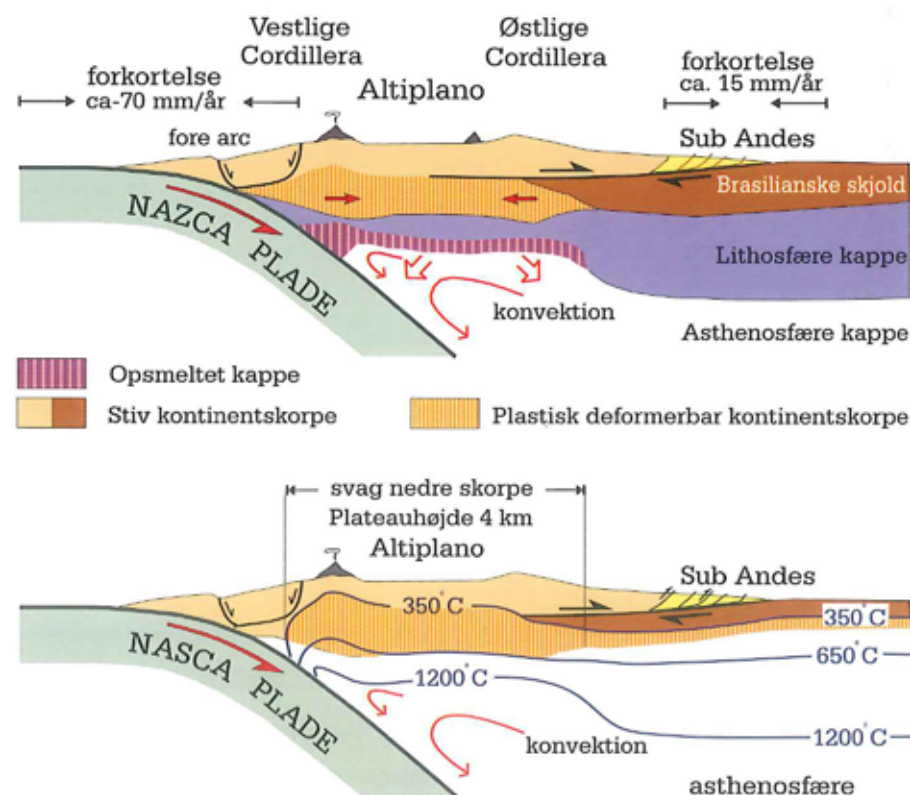
Figur 4. Diagram der illustrerer den formodede litosfærestruktur i Centralandes ved det nordlige Bolivia og Chile. Et Ø-V orienteret profil ved 20° S viser placeringen af den subducerende Nazca Plade og strukturen af den overliggende Sydamerikanske Plade. Øverst: Mægtigheden af den sydamerikanske litosfære er delvist baseret på en fortolkning af helium data og topografi. Nederst: Diagram som skematisk viser de formodede termale strukturer. 350°C isotermerne formodes, at bestemme placeringen af overgangen mellem stiv og plastisk deformation i skorpen. Grænsen menes at ligge langt inde i skorpen under arken og Altiplanoet, samt den vestlige margin af Den Østlige Cordillera, hvor det er muligt at den øvre skorpe flyder på den bløde nedre skorpe. Fra: Lamb & Hoke [1997].
