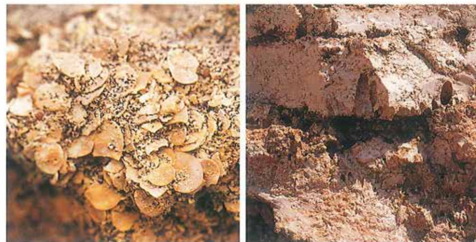
Figur 7. Venstre: Grønsand med linsestore foraminiferer. Il Gelmus, Gozo. Højre: Øvre koralline kalksten. Koral- og algerev boret af daddelmuslinger. Boringerne er ca 12 cm lange. Tat Tomna, Nord-vest Malta.
