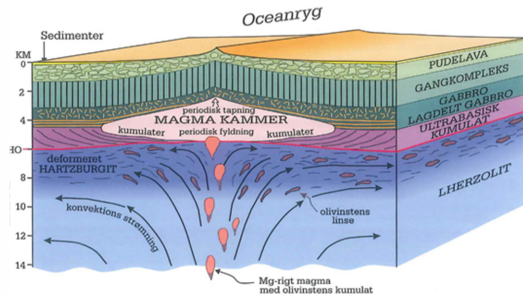
Figur 13. Blokdiagram der viser en model for den tredimensionale opbygning af den øvre kappe og skorpen under en oceanisk spredningsryg, med en skematisk angivelse af de processer, der fører til dannelse af skorpebjergarterne.
