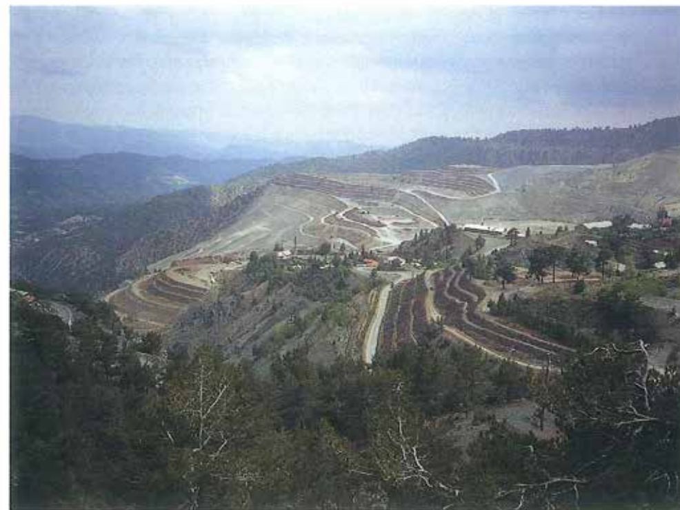
Figur 12. Billede af det åbne brud ved asbestminen nær Mount Olympus centralt i Troodos komplekset. Brydningen er foregået ved afrømning af malmen i terrasser, der tydeligt ses på billedet. Minens dimensioner på overfladen er ca. 1,5 x 2,0 kilometer.
