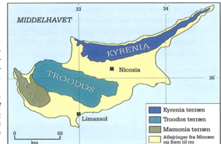
Figur 4. Geologisk skitse-kort af Cypern med de tre geologiske 'terræner', der danner baggrund for Troodos ofiolitkompleksets dannelse. Et geologisk 'terræn' er en distinkt tektonisk enhed med en bestemt geologisk historie – se teksten om sammensætningen af de viste terræner.
