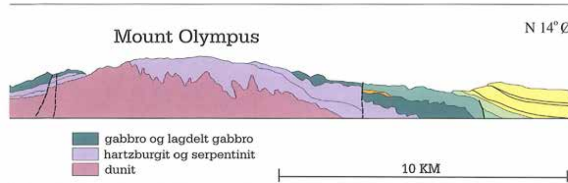
Figur 6. Profilsnit gennem det lagdelte og senere opdømmede Troodos kompleks..
