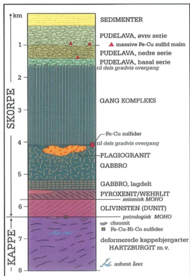
Figur 7. Idealsnit der viser opbygningen af lagserien i Troodos komplekset.
