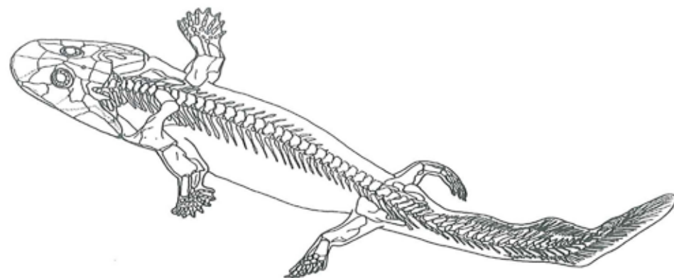
Figur 7. Acanthostega ifølge de nyeste rekonstruktioner. Ribbenene er meget små og hvirveltæppene i ryggraden er meget dårligt udviklet, hvilket gør ryggen meget blød og sandsynligvis ikke i stand til at understøtte dyret på land. Halen er forsynet med store finnestråler, der har båret en stor fiskelignende hale
