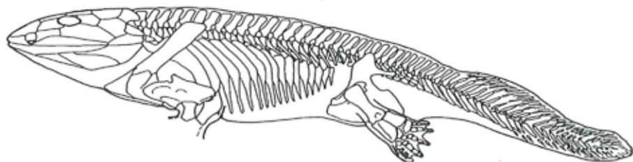
Figur 6. Den nyeste rekonstruktion af urpadden Ichthyostega hvor bagbenene er bagudvendte luffer, hvilket giver Ichthyostega en næsten sællignende fremtoning. De kraftige overlappende ribben har gjort kroppen meget robust og ikke tilladt den store fleksibilitet. Oversiden af halen er forsynet med finnestråler til at bære en halefinne.
