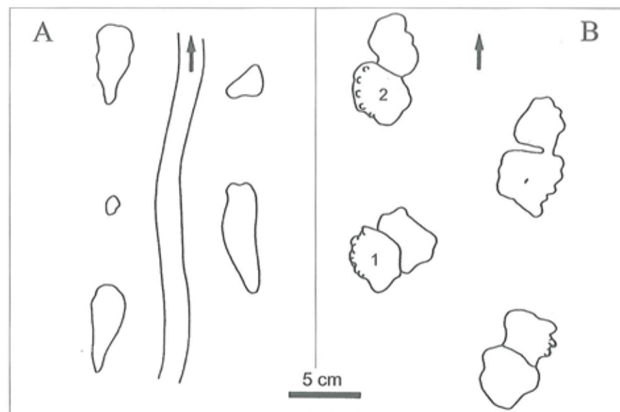
Figur 5. To af sporserierne fra Genoa River, Australien. A: sporserie med lange slæbende aftryk fra bagfødderne og små aftryk fra forbenene. Imellem sporene løber et tydeligt slæbespor fra kroppen eller halen af dyret. B: sporserie hvor aftrykkene af bagfødderne delvist overlapper de mindre aftryk fra forfødderne. I sporene kan skelnes aftryk af mindst fem tæer. Pilene viser bevægelsesretningen
