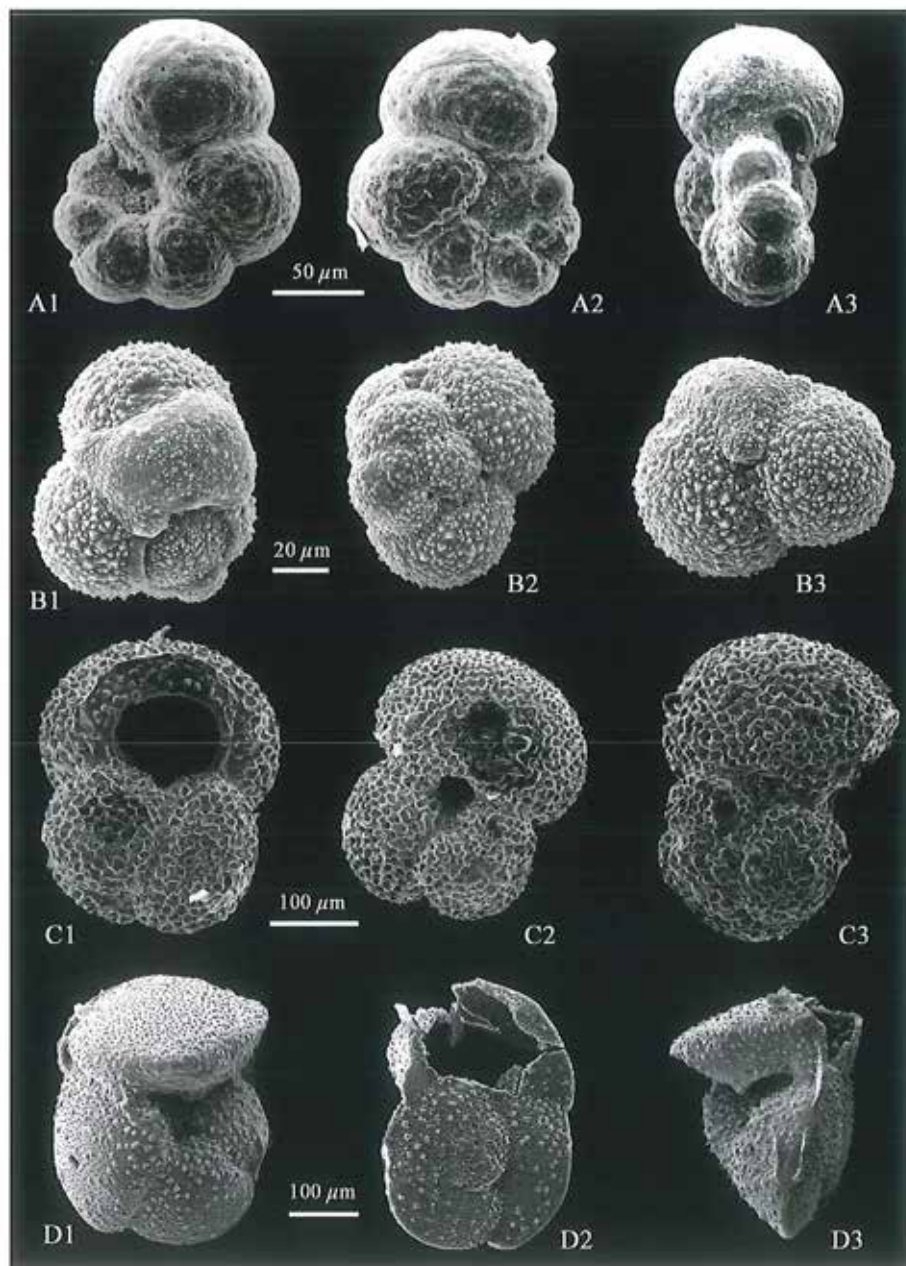
Tavle 6. Udvalgte Globigerinider A1-A3: Berggrenia praepumilio. B1-B3: Globigerinita glutinata. C1-C3: Globigerinoides ruber. D1-D3: Globorotalia truncatulinoides
