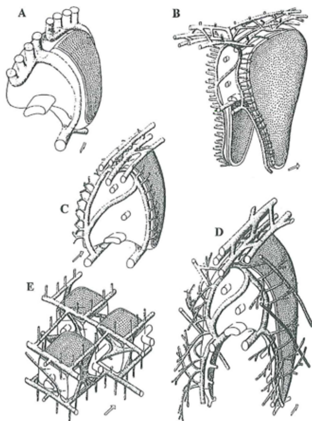
Figur 13. Forskellige typer af kanalsystemer hos (A) Sulco-perculina, (B) Ranikotalina, (C) Operculina, (D) Nummulites og (E) Heterocyclina.
