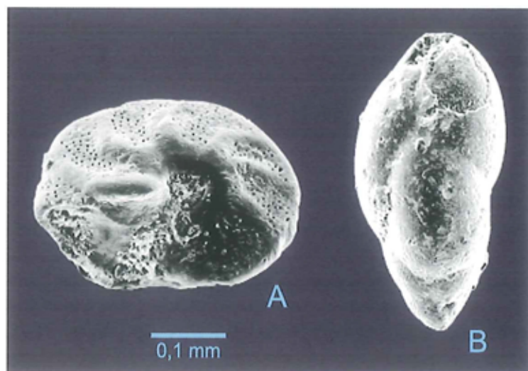
Fig. 1. To typiske skalformer benyttet ved udregning af iltindekset. A: Planokonveks, kalkskallet, bentisk foraminifer almindelig under velilteede forhold. Torpedoformet, kalkskallet, bentisk foraminifer, tolerant over for dårligt iltede forhold.
