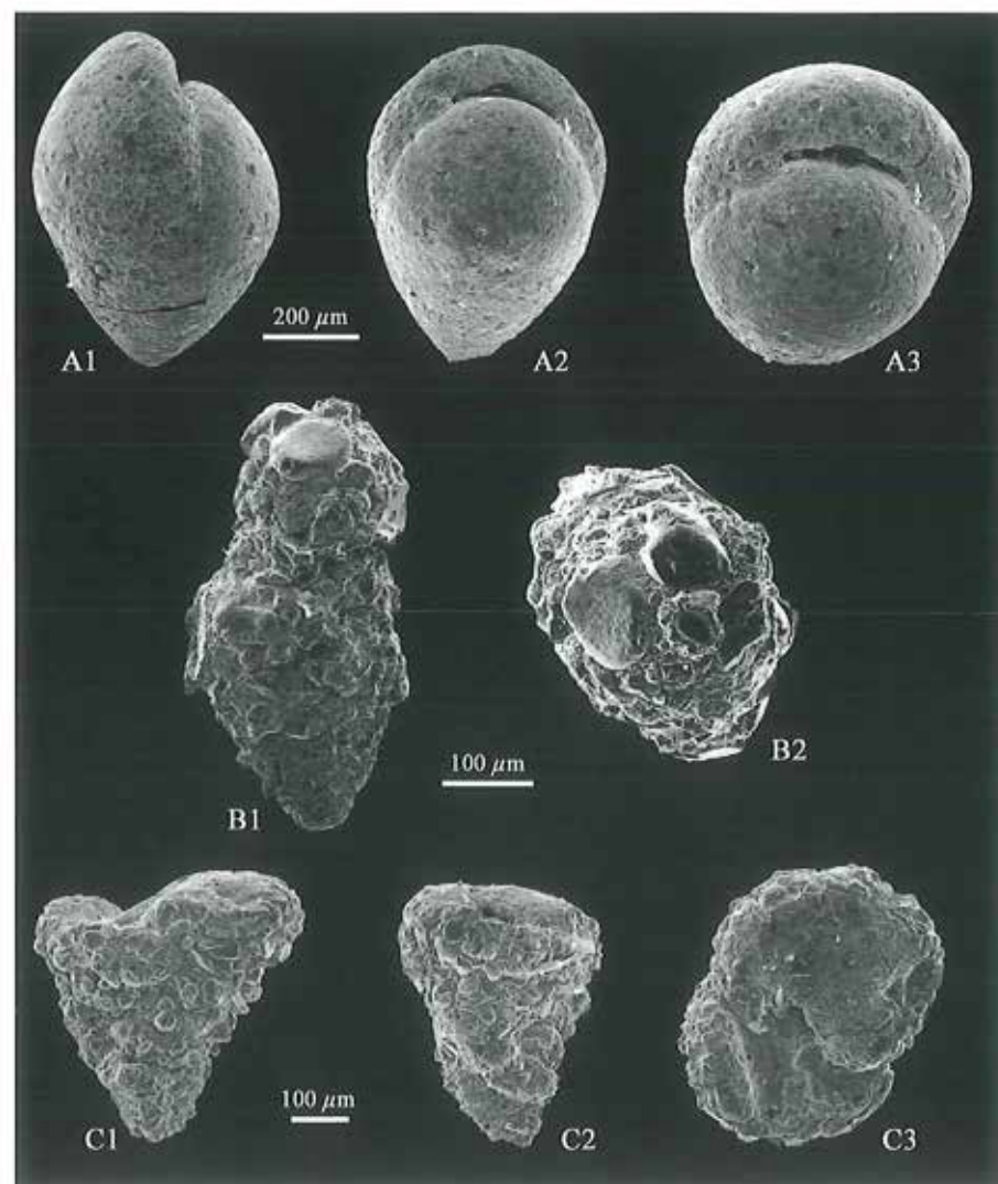
Tavle 2. Udvalgte agglutinerende foraminiferer.
