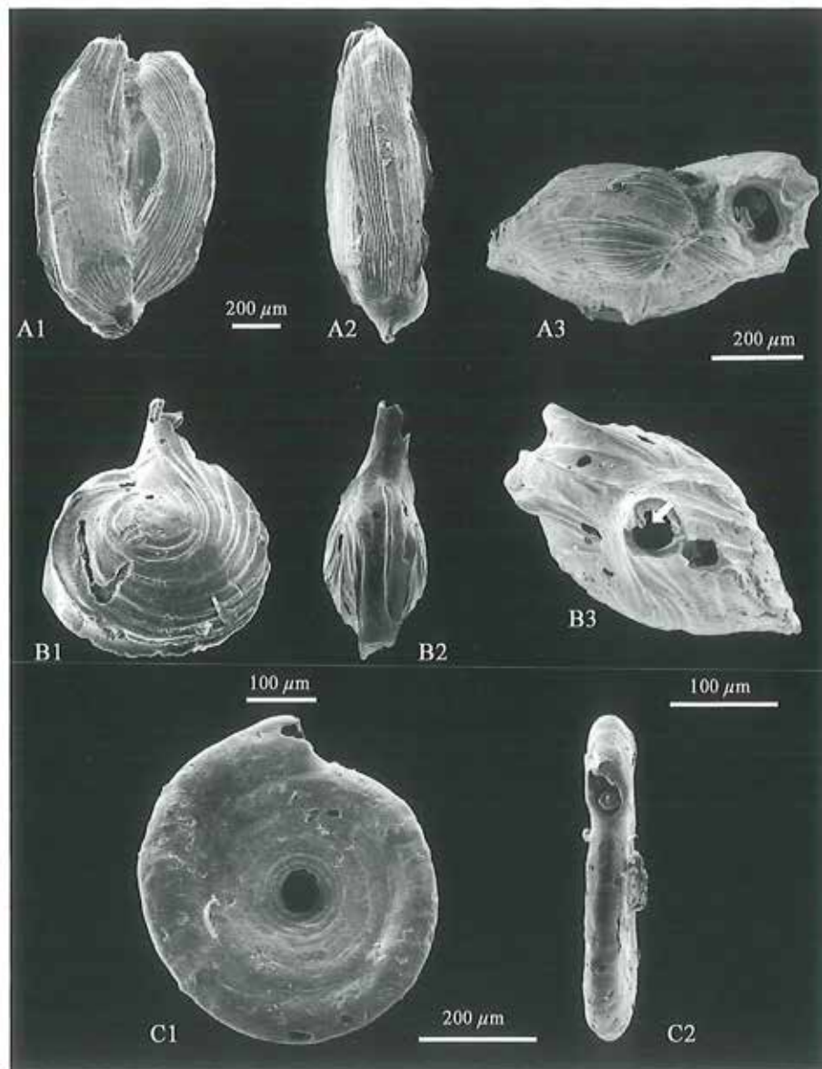
Tavle 3. Tre udvalgte Milionider
