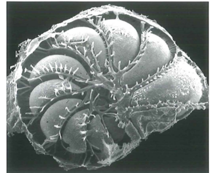
Figur 12. Afstøbning af Rotalioid foraminifer.
