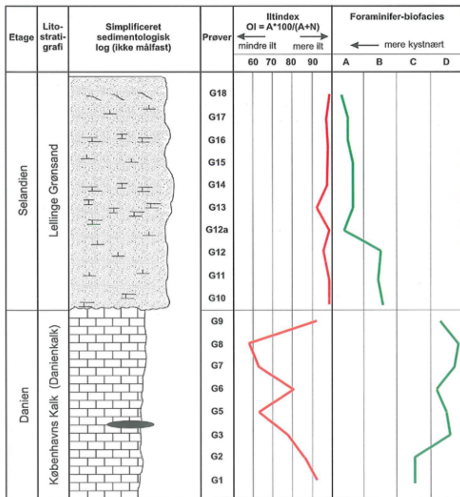
Fig. 3. Skematiseret, sedimentologisk log med angivelse af iltindeks og biofacies for hver af de analyserede prøver. Kurverne viser, at de mest velilte forhold - ikke overraskende - findes i de mest kystnære aflejringsmiljøer.
