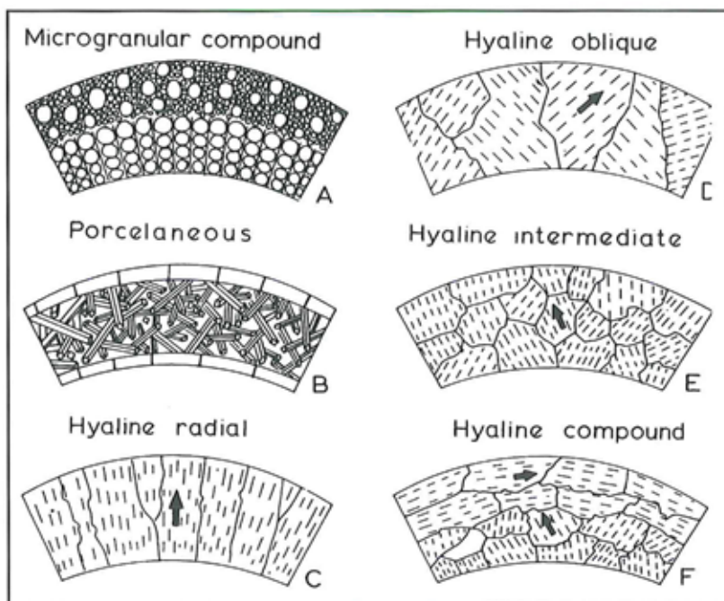
Figur 3. Skålvægskrystalstruktur hos (A) de mikrogranulære, (B) de porcelænsagtige og (C-F) de hyaline. Pilene viser orienteringen af krystallernes C-akse, se tekst.
