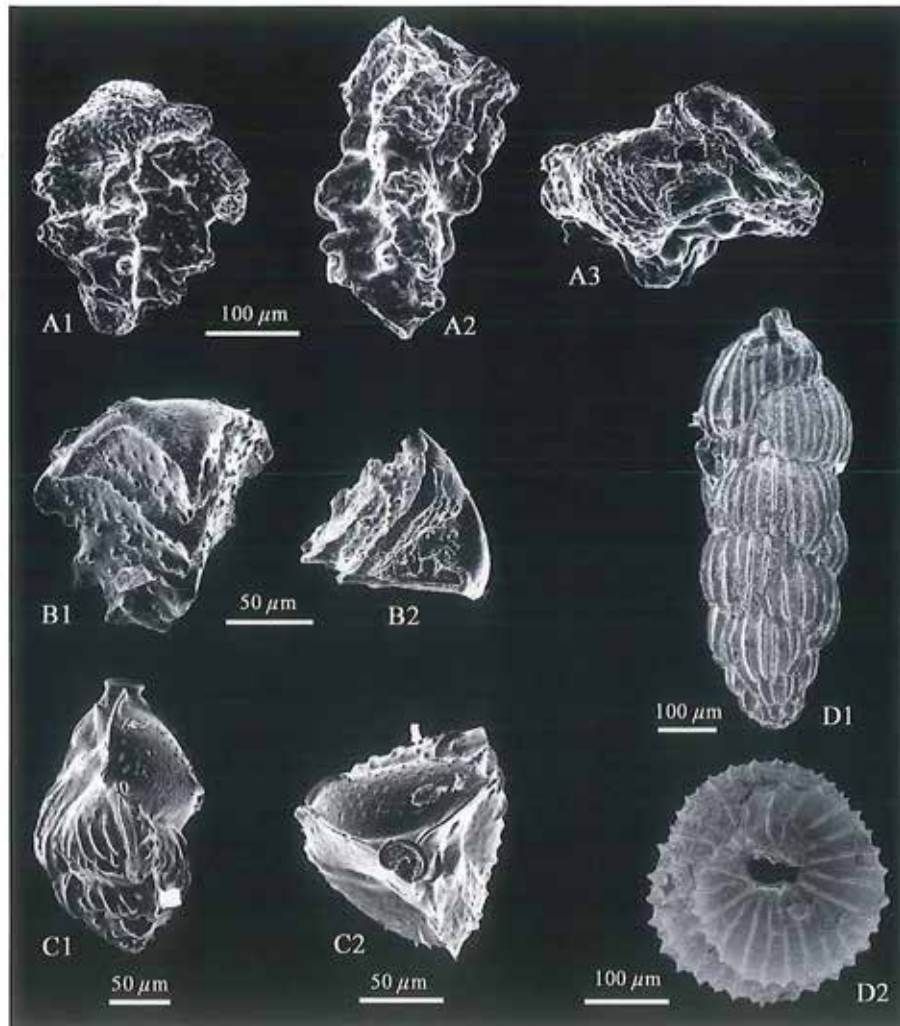
Tavle 8. Udvalgte bulliminider A1-A3: Bolivina plicatella. B1-B2: Reusella spinulosa. C1-C2: Trifarina angulosa. D1-D2: Uvigerina peregrina
