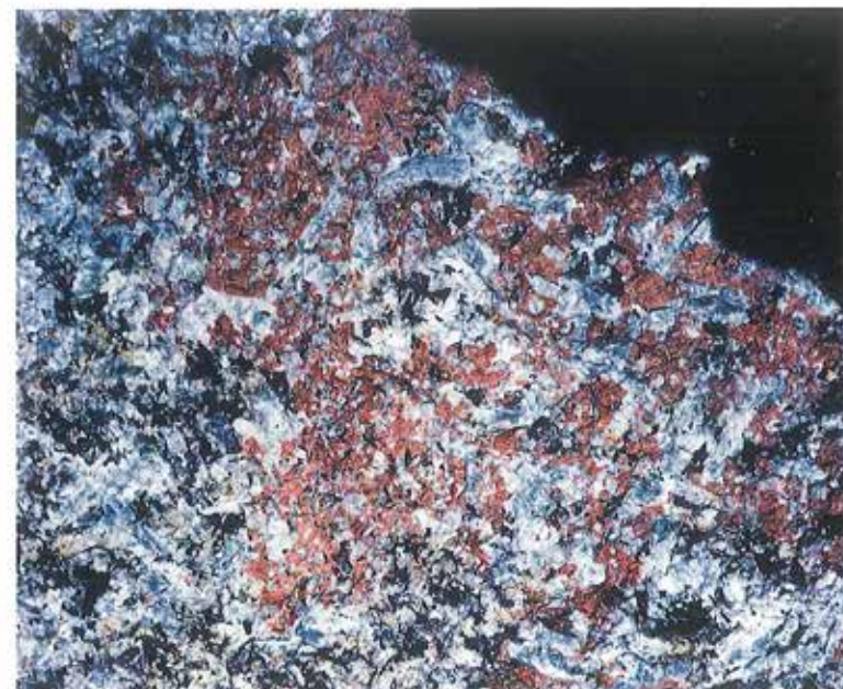
Bjergarten naujait fra Ilimaussaq-komplekset i Sydgrønland. Små grønne korn af mineralet sodalit er indlejret i store korn af mineralerne hvid feldspat, rød eudialyt og sort arfvedsonit og ægirin.
