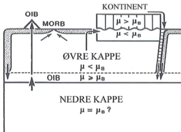
Figur 4: Skematisk diagram der viser de kappe- og skorpereservoir, der er relevante for blyisotopstudier. OIB = Ocean Islands Basalts, MORB = Mid Ocean Ridge Basalts. \mu = reservoirs nuværende ^{238}\text{U}/^{204}\text{Pb} -forhold, \mu_B = ^{238}\text{U}/^{204}\text{Pb} af den totale Jord.
