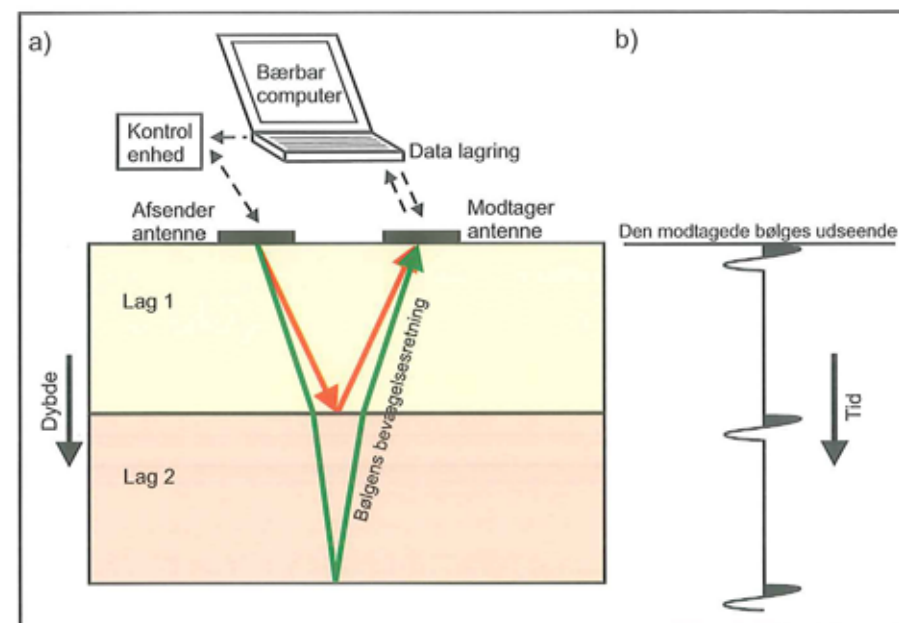
Figur 2. Principskitse af (a) en georadarooptagelse og (b) billedet af den registrerede elektromagnetiske bølge, hvor udsvinget på linien viser, at jordens elektromagnetiske egenskaber ændres ved grænsen mellem lag 1 og lag 2.
