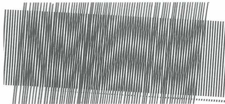
Et moirémønster fremkommet ved, at to lidt forskelligt orienterede sæt af parallelle linier er lagt over hinanden. Mønstret ændrer sig med vinkelen mellem linierne.
