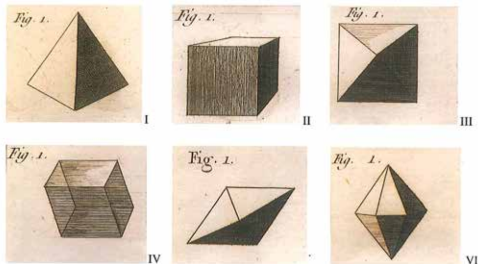
Figur 2. Romé DeLisle's 6 grundformer. I tetraeder, II terning, III det retvinklede - dvs. kubiske- oktaeder, IV det rhomboidale parallelipedum, dvs. vort trigonale rhomboeder, V det rhomboidale oktaeder, dvs. vor orthorhombiske bipyramide, VI dodekaedret med trekantede flader, dvs. vor hexagonale bipyramide.
