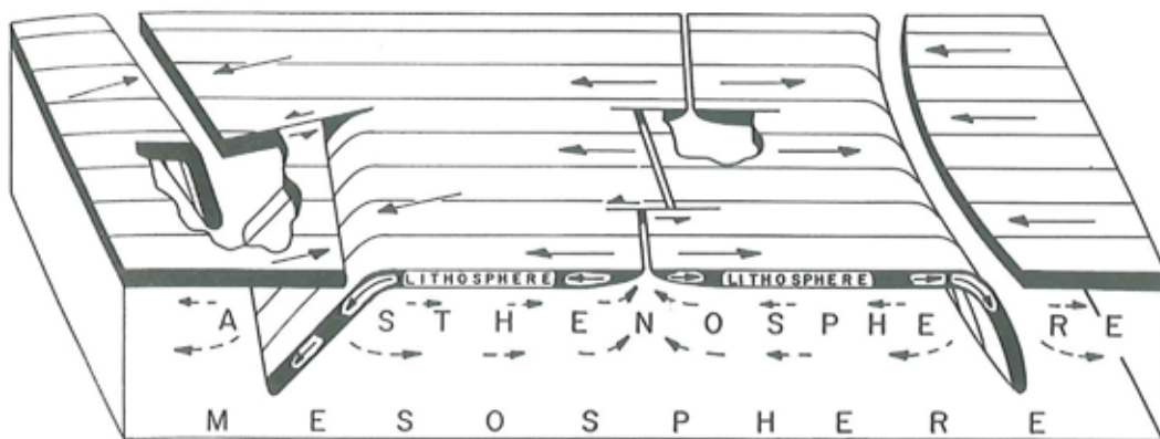
Skematisk blokdiagram som viser en pladetektonisk model. Lithosfæreplader bevæges væk fra en oceanryg, som er forsat af to transforme forkastninger. Lithosfærepladerne føres nedad i subduktionszoner med dybgrave og øbuer, til højre en simpel øbue, til venstre en øbue som er forsat af en transform forkastning. Konvektionsstrømme i asthenosfæren kompenserer for den nedadrettede bevægelse af lithosfærepladerne (efter B. Isacs, J. Olivier og L.R. Sykes 1968).
