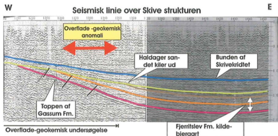
Figur 4. Figuren viser en seismisk linie over den østlige flanke af Skivestrukturen. Lagdelingen er angivet med farvede linier. Den geokemiske anomali i området synes relateret til forkastningsblokke på Gassum niveau, idet Gassum blokkene ligger under den geokemiske anomali.
