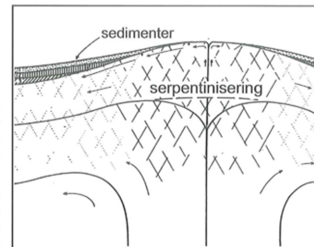
Diagram der viser konvektionsstrømme som stiger op under en oceanryg og bevæger sig ud til siderne, hvorved også den overliggende skorpe bevæges væk fra ryggen. Denne bevægelse væk fra ryggen bekræftes af at oceanbundssedimenterne overlapper hinanden og bliver yngre ind mod ryggen. Fundet af blokke af serpentiniseret peridotit nær ocean-ryggene fik Hess til at foreslå at den nederste del af oceanskorpen består af dette materiale (efter Harry H. Hess, 1962).
