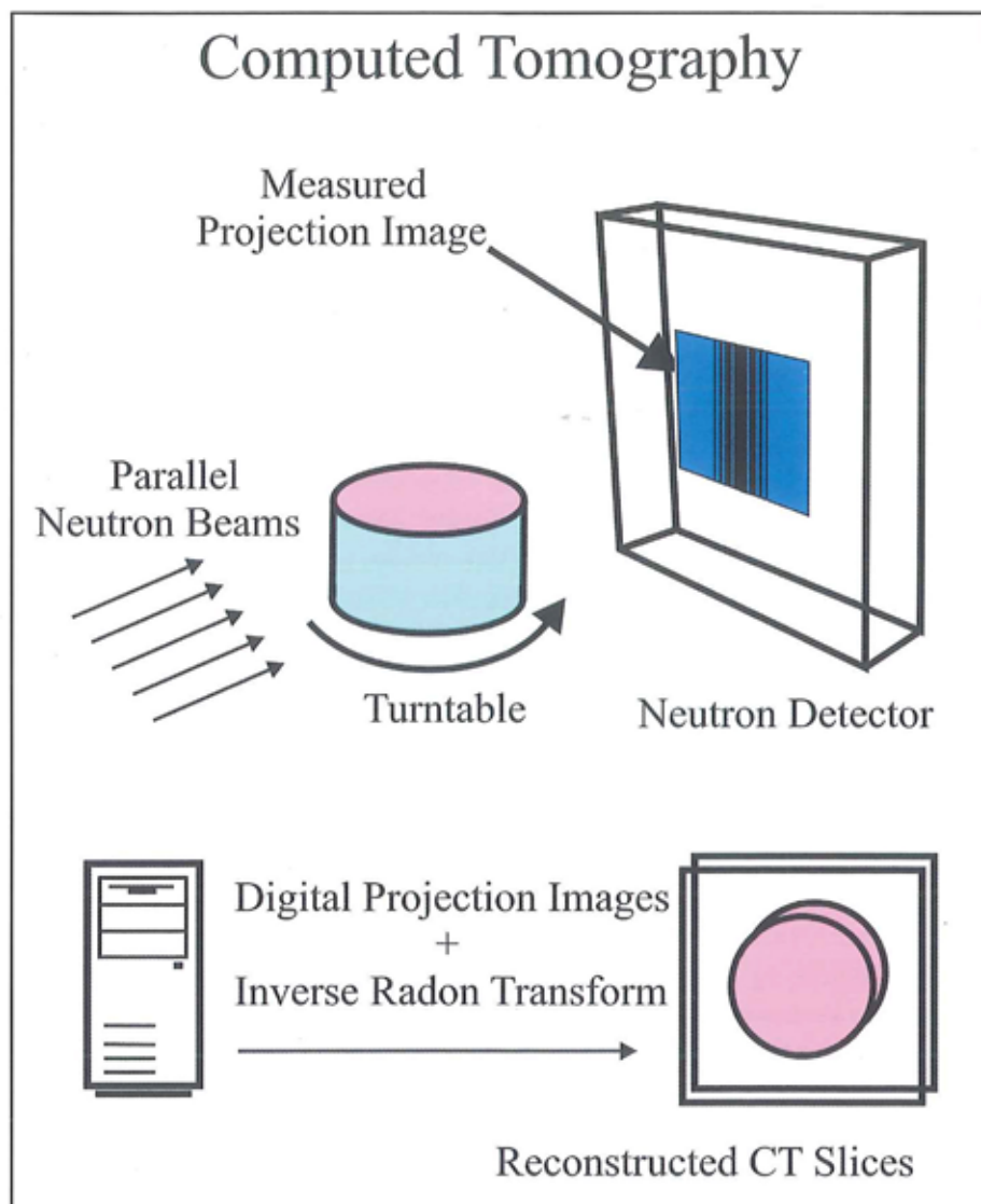
Figur 4. Princippet bag neutrontomografi taget fra Paul Scherrer Institutet (PSI's) hjemmeside. Neutronstrålen kommer ind fra venstre, gennemlyser prøven, og der optages et billedet på en to-dimensional detektor. Prøven drejes en smule og processen gentages som regel flere hundrede eller tusinde gange. Den tre-dimensionale struktur kan derefter rekonstrueres med hjælp af rekonstruktionsalgoritmer og rå computerkraft.
