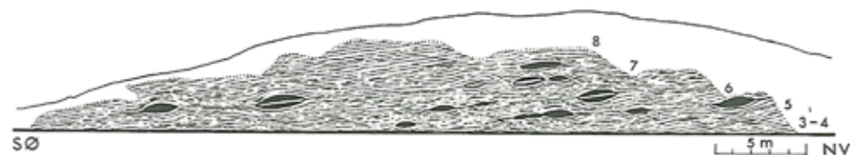
Figur 9. Profil i Olenid-skiferen (øvre kambrium) ved lokalitet 27, Læså.
