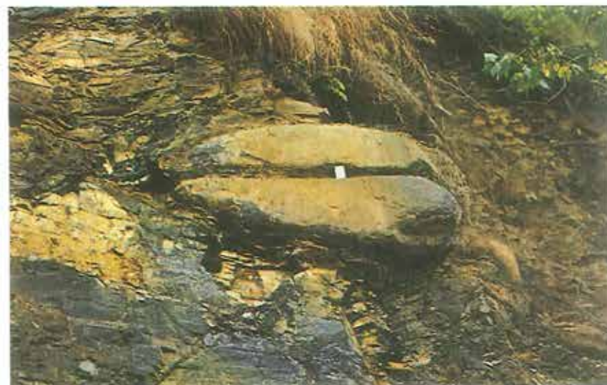
Antrakonit-bolle i Olenid-skiferen ved lokalitet 27. Det gullige overtræk på skiferen og antrakonit-bollen er udskilt kalium-jernsulfat. Cigaretten i midten af billedet er godt 5 cm høj. VP.fot.
