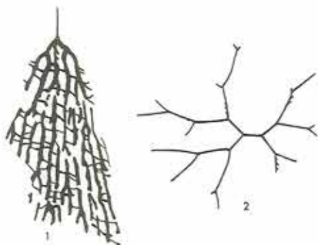
Figur 12. Graptoliter fra Dictyonema-skifer (ældste ordovicium). 1: Dictyonema, 2: Clonograptus.
