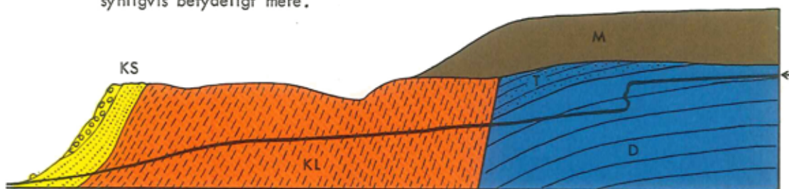
Figur 18. Profil af lagene ved Risebæks munding. D = Dicellograptusskifer, T = Tretaspiskifer, KL = keuperler, KS = keupersand og konglomerat. M = moræne. Pilen peger mod bæklobets bund.
