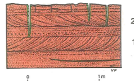
Figur 16. Skematisk snit i Nexø Sandsten. 1 og 2 krydslejrrede lag afsat af strømmende vand fra henholdsvis højre og venstre.
