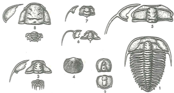
Figur 24. Trilobiter fra 'Olenid Skiferen'. 1: Olenus (Øleå), 2: Agnostus (Øleå), 3: Parabolina, 4: Orusia, 5: Eurycare, 6: Ctenopyge, 7: Sphaerophthalmus, 8: Peltura.
