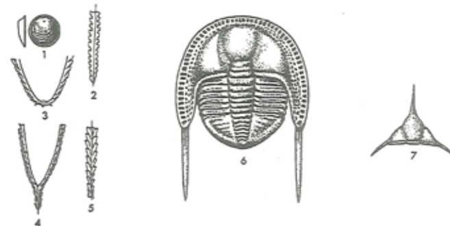
Figur 26. Fossiler fra 'Dicellograptus Skifer' (1-5) og 'Tretaspis Skifer' (6-7). 1: Paterula (brachiopod), 2: Climacograptus, 3: Dicellograptus, 4: Dicranograptus, 5: Diplograptus, 6: Tretaspis, 7: Lonchodomas.
