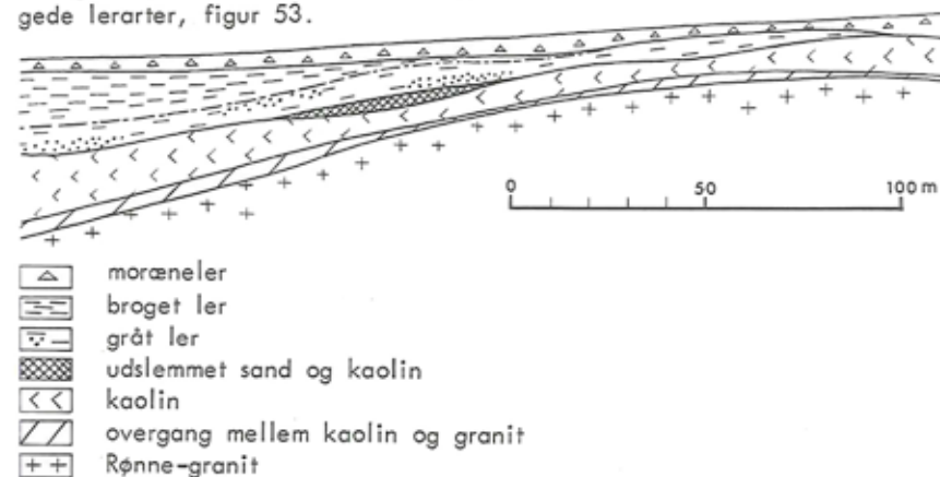
Figur 53. Snit gennem lagene ved Rabekkeværket. (P.Graff-Petersen og J.Bondam).
