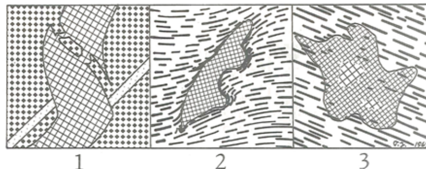
Signaturer: Stribet: gnejs - sorte kvadrater: granit - prikker: aplit - kvadratnet: leukogranit og pegmatit.
