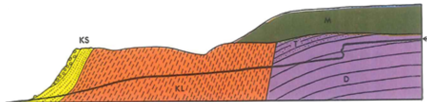
Figur 34. Profil af lagene ved Risebæks munding. D = 'Dicellograptus Skifer', T = 'Tretaspis Skifer', KL = Keuperler, KS = Keupersand og konglomerat. M = moræne. Pilen peger mod bæklobets bund.
