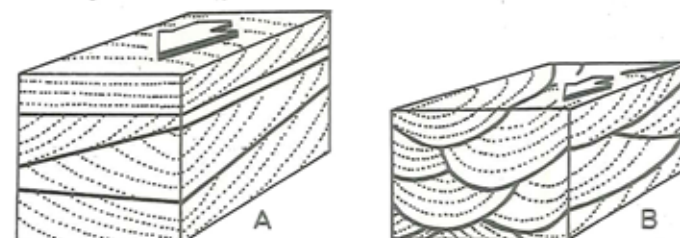
Figur 45. Storskala planar krydslejring (A) og storskala trugkrydslejring (B). De optrukne streger viser begrænsningen af et lag. De stiplede antyder orienteringen af de frontlejrte smålag inden for laget. (Omtegnet efter Blatt, Middleton og Murray).
