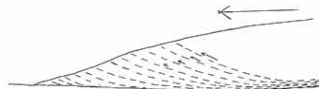
Figur 67. Snit gennem en gletscher, der viser, hvorledes islager glider frem over hinanden og hælder mod gletscherbevægelsen. Bevægelsen er mindst i bunden af gletscheren.
