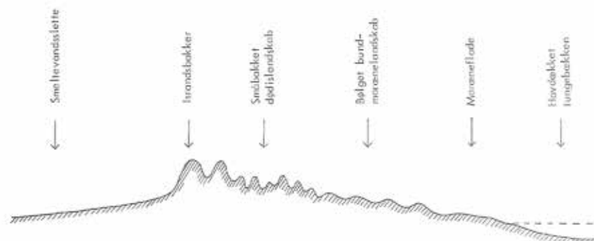
Figur 63. Snit gennem glacial landskabsserie.
