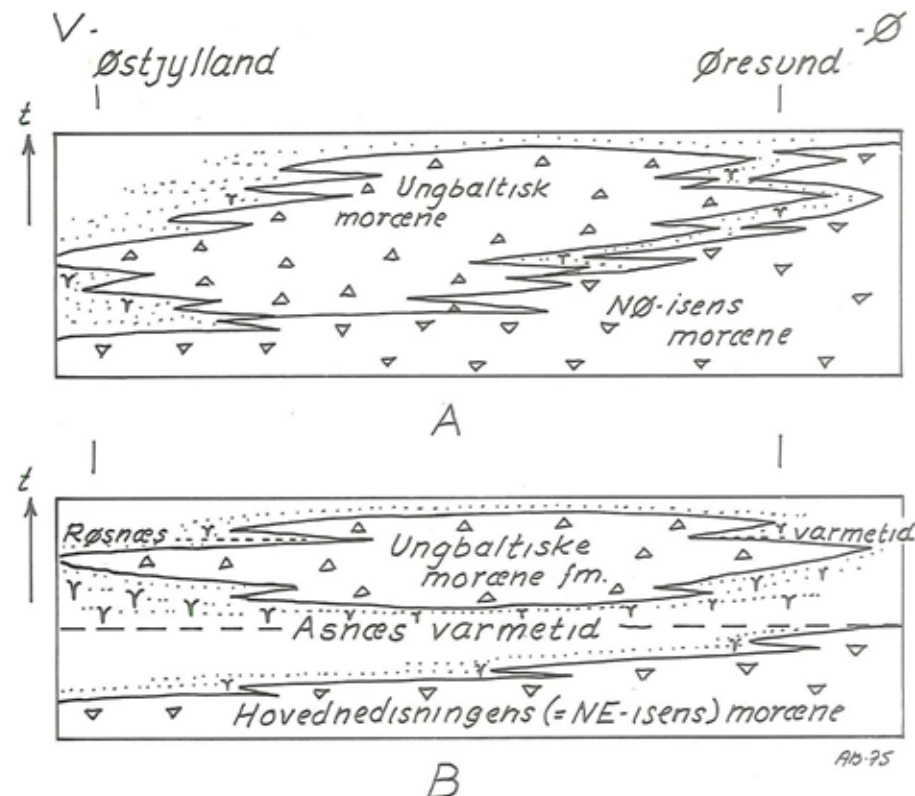
Stratigrafiske modeller for Weichsel istidens afsmeltningstadiet. I model A er der interferens mellem NØ-isen og den Ungbaltiske is. B er en model med klart tidsadskilte fremstød.
