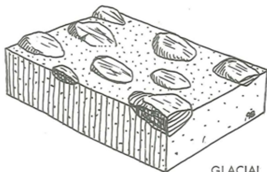
GLACIAL BROLÆGNING
