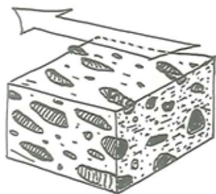
a-PRÆGET STENORIENTERING
