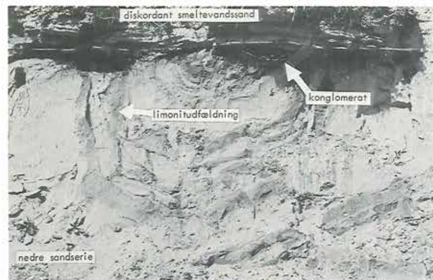
SKALFORMET LIMONITKONKRETION FRA ASNÆS VARMETIDEN, LOSSEPLADSEN VED ULSTRUP.
