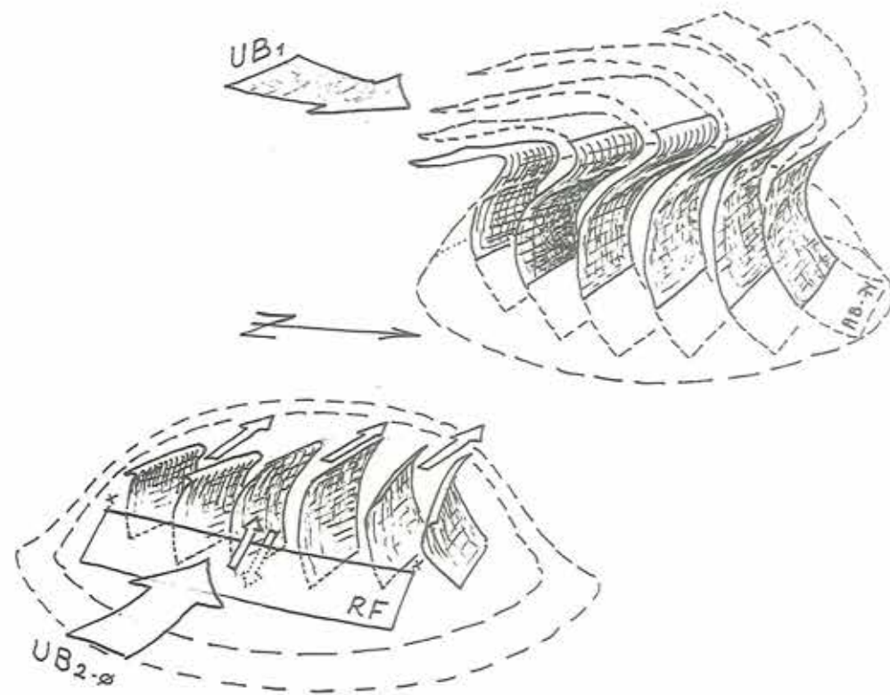
Principskitse af Store Ulvebjerg. Øverst ses sand- og gruslagene opskudt af istryk fra SV (første Ungbaltiske fremstød). Nederst ses de foldede lag at blive ombøjet i bakkens top som følge af medslæb ved isoverskridelse fra ØSØ-lig retning. RF angiver orienteringen af opskydningsforkastninger.
