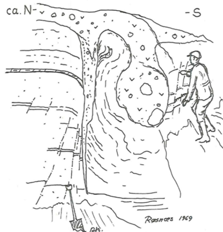
Iskilestruktur gennemgående en vasestruktur i grusgraven ved Næbbedynd. Bemærk at iskilestrukturen skærer vasestrukturens deformerede sandlag i den nordlige del af profilet.
