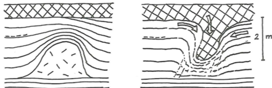
Rekonstruktion visende, hvorledes en vasestruktur kan dannes ved udsmelting af et klokkeformet islegeme. Det skraverede lag er moræneler. Sammenlign med figuren side 22. Pilene angiver indflydningsbevægelsen under udsmeltingen.
