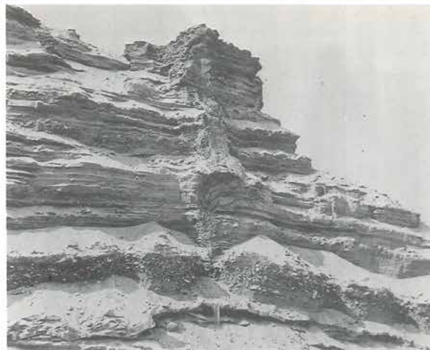
KILE-I-KILE STRUKTUR I ØVRE LAGSERIE. STENSBJÆRG.
