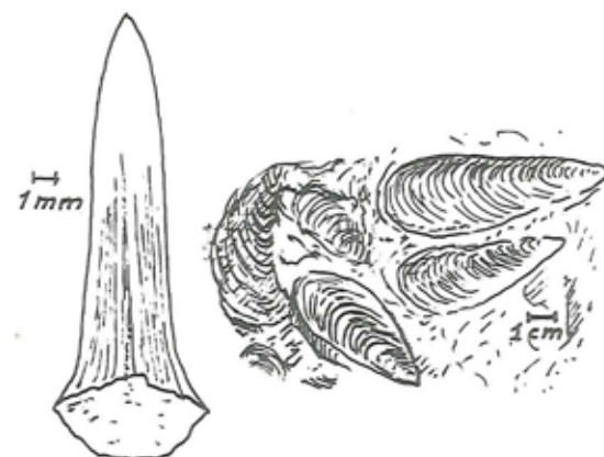
Nedre Eocæn højtand og brudstykke fra konkretion med Mytilus roenaeensis nov.sp. (efter Petersen m.fl. 1973).
