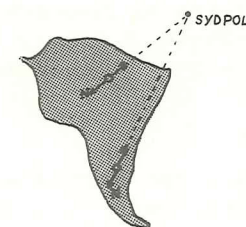
5. Position af sydpol i Devontiden, beregnet ud fra Devon-bjergarter i Sydamerika.
