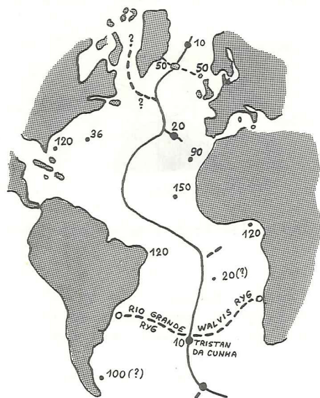
3. De atlantiske vulkaners alder (efter Nature).
