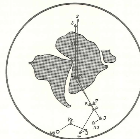
7. "Polvandrings"-ruter ved sammenskydning af kontinenterne. Kun Afrika og Sydamerika er indtegnet. (efter Nature)
