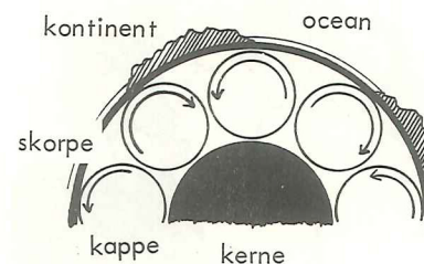
1. Forholdet mellem kontinenter og konvektionsceller.
