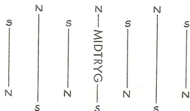
4. Magnetstyrker ved den midtatlantiske ryg.
