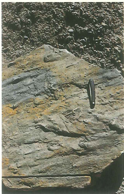
Flysch-lagflader
