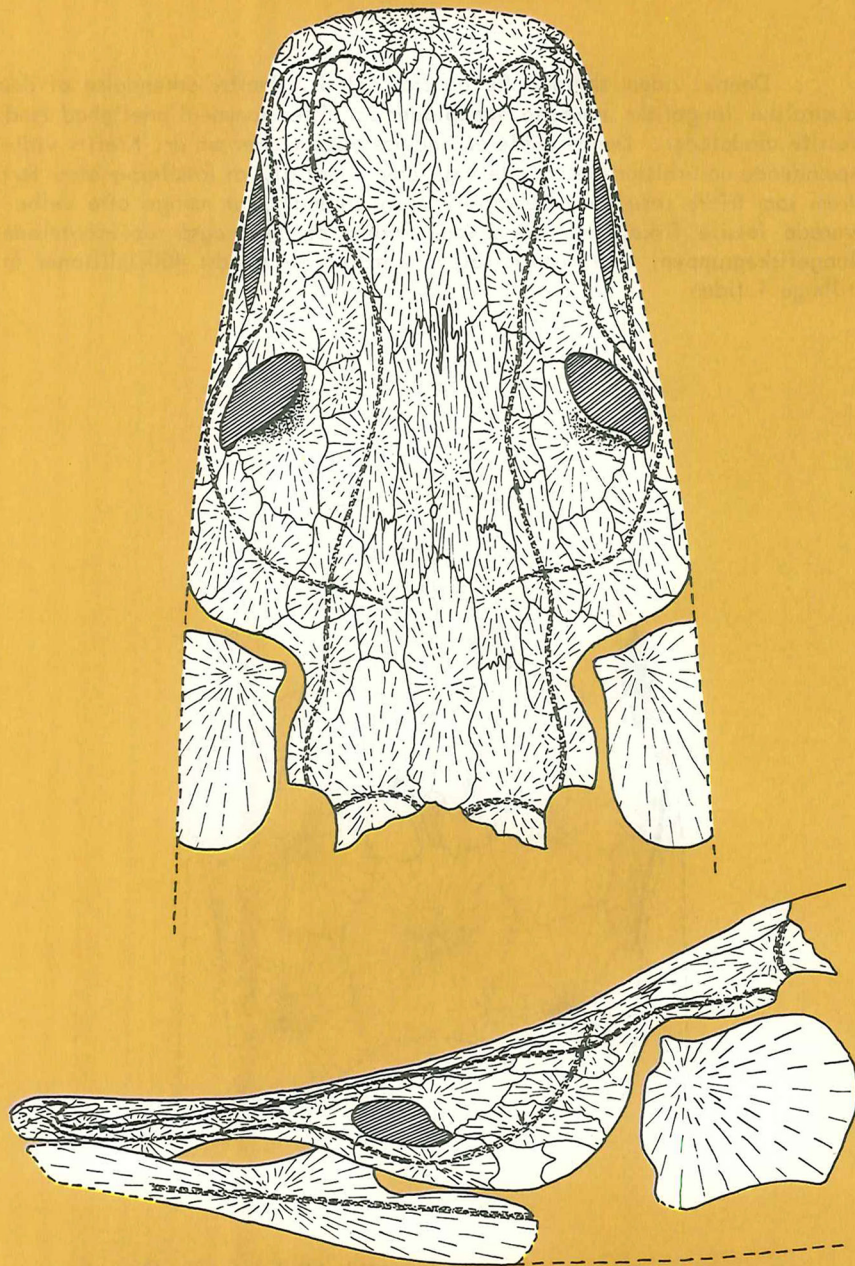
Rekonstruktion af den langsnuddede lungefisk Soederberghia (set oppefra og fra siden). Øvre devon, Østgrønland. (Efter Lehman 1959).
