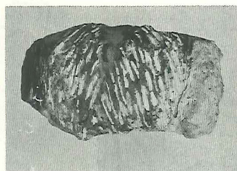
Forstenede lungefiske-køkon'er i lerskifer-aflejringer fra Texas nedre perm. Derunder ses opspaltede dele af sådanne køkon'er med skeletrester af lungefisken Gnathorhiza , der er en meget nær slægtning til de nutlevende afrikanske og sydamerikanske lungefisk.
