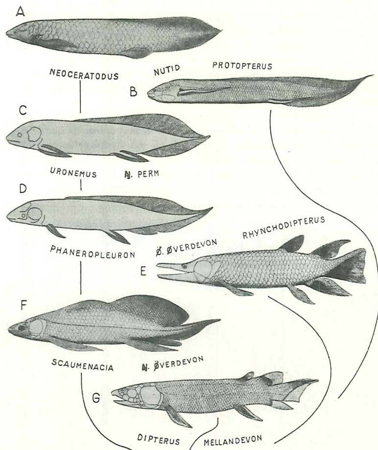
Lungefiske-gruppens vigtigste udviklingslinier illustreret gennem godt kendte fossile former fra devon- og perm-tiden samt de nu-levende australske og afrikanske repræsentanter. (Efter Jarvik 1959).
