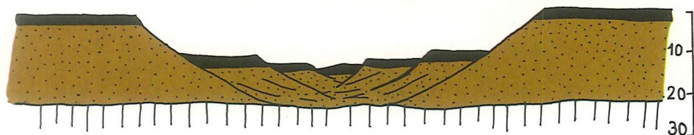
Figur 8. Snit på tværs af Langdalen med angivelse af skredstrukturer fremkommet ved udskridning langs 30° hældende forkastningsplaner. De enkelte større blokke eller "kulisser" vil næppe bevare deres indre struktur. De vil efterlade en ujævn dalbund med langstrakte rygge i dalens længderetning. Sådanne former kan netop iagttages enkelte steder i Langdalen.
