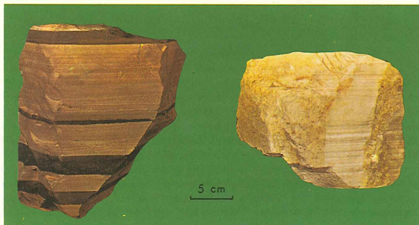
Til venstre: Cementsten (kalkkonkretion) med askelagene +27 (nederst) til +30, der er et "dobbeltag" det vil sige to askelag lige oven på hinanden. Til højre: Egentlig moler, en lys diatomit uden kalk. Begge sten viser den fine laminering med skiftende tynde, lyse og mørke lag.
