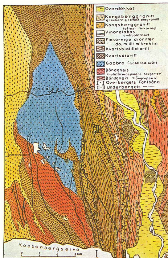
Geologisk kort over Kongsbergfeltet. Kvarts-breccieårer og sølvførende kalkspatårer er ikke indtegnet.
