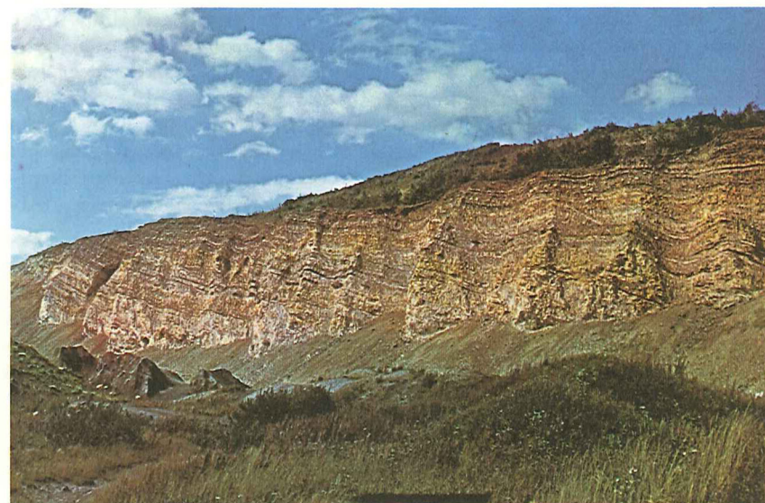
Nordvæggen af den forladte, nordlige molergrav ved Færkør, til venstre ses en rest af de mørke, lerede lag fra molerets nedre del, mens det meste af brydningsafsnittet er bortgravet, og askeafsnittet står tilbage.
