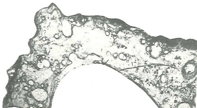
Figur 2. Udsnit af væggen af lynørret i figur 1 set under stor forstørrelse. Vægtykkelsen er 1 mm. Glasmassen fremtræder som strukturløs, glasboblerne er hvide og afrundede. I venstre, ydre kant ligger et ikke-smeltet feldspatkorn (foto M.Ghisler).
