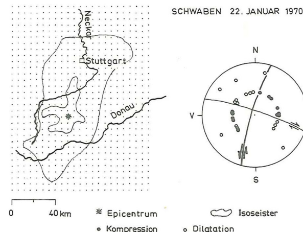
Figur 7. Jordskælvet i Schwaben 1970. Til venstre: kort over placeringen af epicentrum. Bemærk NNØ-SSV udstrækningen af isoseisterne. Til højre: beregning af forkastningens retning ud fra retningen af primærbølgerne første pulsslæg på seismograferne.
