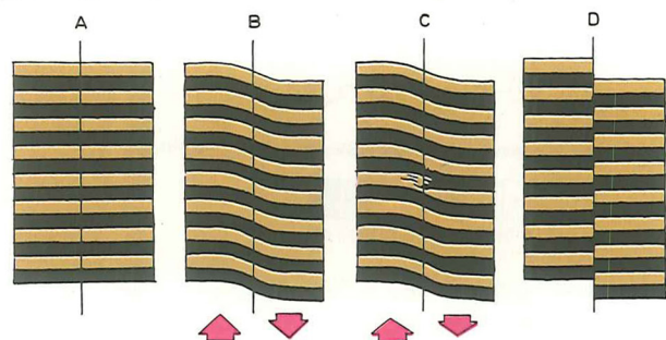
Figur 5. Deformation og forskydning resulterende i jordskælv-forskydninger kan både foregå i horisontal og vertikal retning. A: strukturel ro. B: deformation. C: pludseligt brud og forskydning som kan udløse jordskælv. D: strukturel ro efter forskydning. (modificeret efter Reid).
