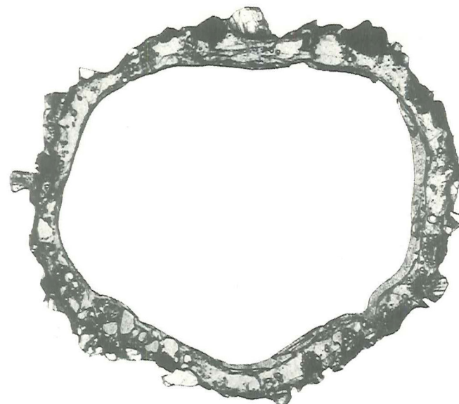
Figur 3. Lyrør fra Herning set i tværsnit. Min.Mus.Saml. Den indre diameter måler 6,5 \times 5,5 mm. Rørets glasmasse er tydeligt tyndere end i lyrerøret fra Lüneburg - 0,5 mm - og det indeholder flere ikke-smeltede mineral Korn. Mikrofoto uden polarisator (M.Ghisler).
