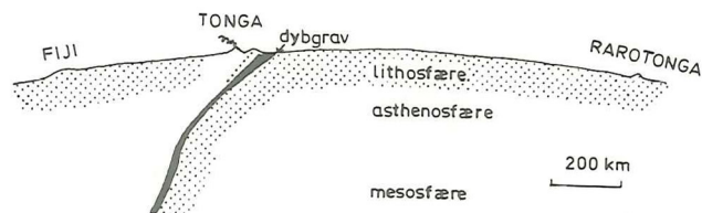
Figur 3. Lodret snit gennem Tonga-dybgraven visende zonen med de dybe jordskælv ("Benioff zonen"). Den dybtliggende jordskælvsaktivitet skyldes, at en jordskorpeplade (fra højre) underskydes og når dybt ned i kappen.
