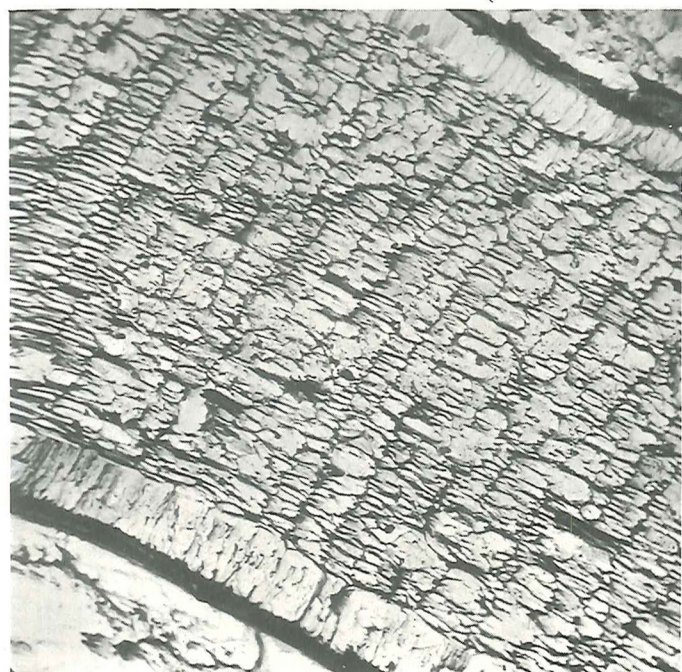
Figur 6. Snit gennem Scaphites-skål. Forstørret cirka 1350 gange.
