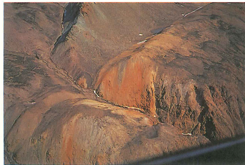
Figur 6. Rhyolit- og tufbjergarter omgivet af Devone sandsten. Rhyoliten, der er beriget på radioaktive grundstoffer, er stærkt rødfarvet på grund af iltning.
