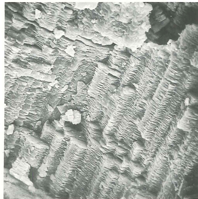
Figur 7. Brudflade af perlemor fra ammonit. Forstørret cirka 1050 gange.
