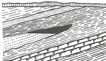
Stratigrafisk olie fælde: olie + gas opfanget i udkilende lag af sandsten i en hældende lagserie af lerskifer.
