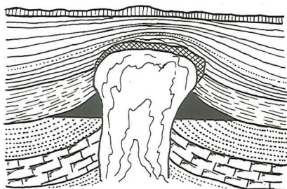
Olie opfanget i opbøjede lag langs salt diapir.
