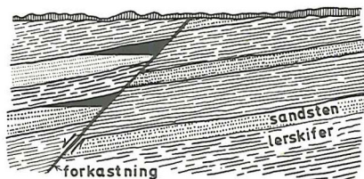
Olie (sort) opfanget i svagt hældende sandsten, hvor denne langs en forkastning er bragt i kontakt med en uigennemtrængelig lerbjergart.
