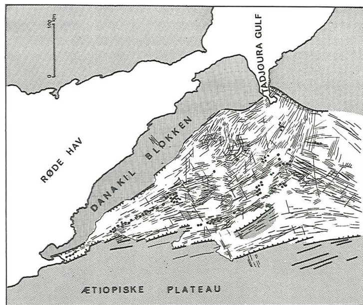
Figur 3. Tektonisk kort over Afar-området med de vigtigste for- og tilbageflytninger. De store riftforkastningszoner er angivet med takker i hældningsretningen. Med prikker er angivet områder med termal aktivitet (vulkaner, varme kilder og gasudstrømningssteder - fumaroler).
