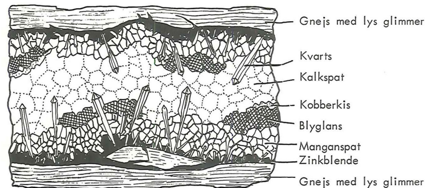
Tværsnit gennem en malmgang, Himmelsfürst-Fundgruben ved Brand, Erzgebirge. Sidestenen er sericitiseret gnejs. I gangen er kvarts ældst, derefter følger zinkblende, manganspat, blyglans, kobberkis og kalkspat. Efter W.Maucher.
