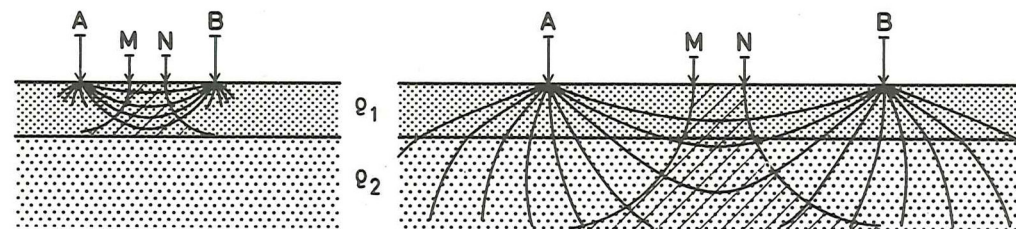
Figur 2. Stigende måledybde med større elektrodeafstand.
