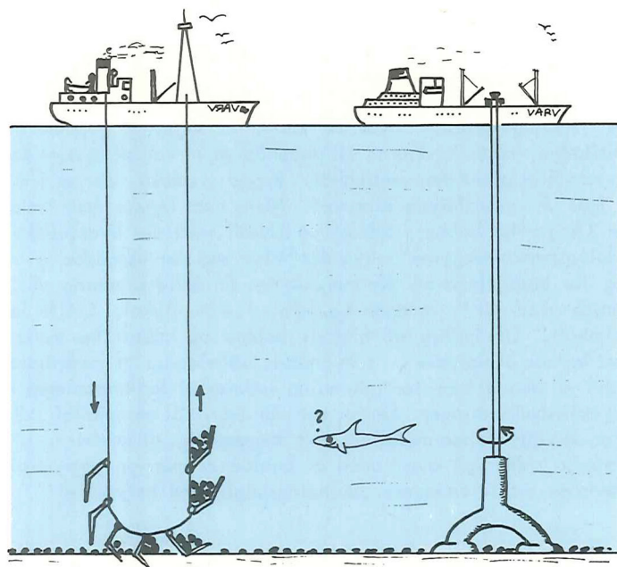
Figur 5. Skematisk tegning af to afprøvede systemer til brydning af manganknolde, til højre det hydrauliske system foretrukket af amerikanerne.
