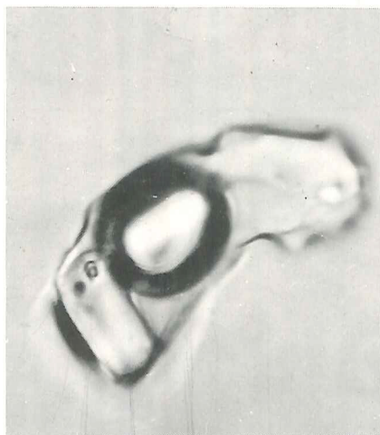
Gas-væske-indeslutning med stensalt og uidentificeret krystal som datter-mineraler.
