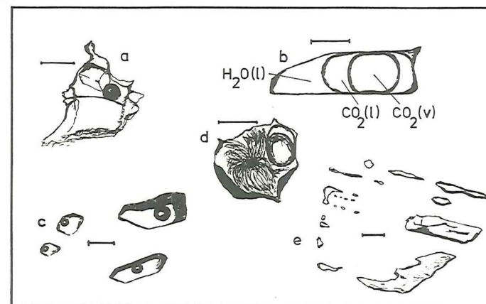
Figuren viser forskellige former for indeslutninger: a) meget uregelmæssig væskeindslutning, med en terning af NaCl. b) rørformet indeslutning med en blanding af \text{CO}_2 og \text{H}_2\text{O} . c) gruppe af små væske-gas-indslutninger. De mindste afgrænses af de samme krystalflader som kvarts ("negative krystaller"). d) samme type indeslutning som b. Her ses desuden "dunet" dateterminal, dawsonit. e) rekrystalliseret sprække med methanindslutninger. Målepinden er 1/20 mm lang.
