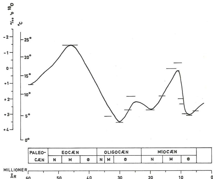
Figur 4. Temperaturvariationerne i Nordsøen gennem Tertiær-perioden på basis af iltisotop-indholdet (skala længst til venstre) i fossile snegle- og muslingeskaller. De vandrette streger viser de enkelte målinger, idet stregens længde er et udtryk for den tilsvarende usikkerhed i aldersbestemmelse.
