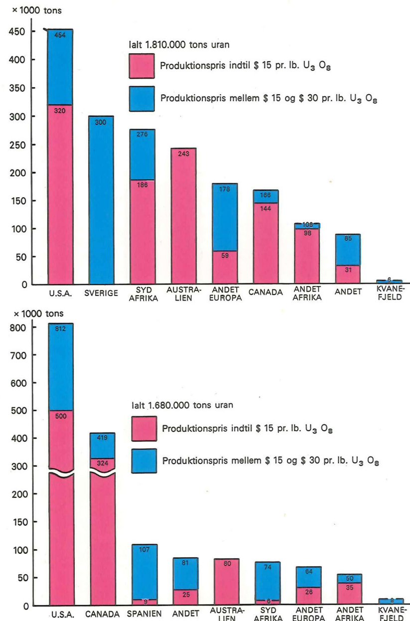
Figur 2. De to sæt søjler viser den vestlige verdens uranreserver, som de var opgjort i januar 1975. Øverst ses de "sikkert bestemte" reserver og nederst de "sandsynlige" reserver. Uranforekomsten på Kvanefjeldet i Sydgrønland er tegnet ind på figuren, selvom det endnu ikke er vist, at produktionsprisen kan holdes under 30$ per lb U_3O_8 .
