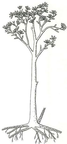
Figur 13. Rekonstruktion af Glossopteris træ (efter D.Pant).
