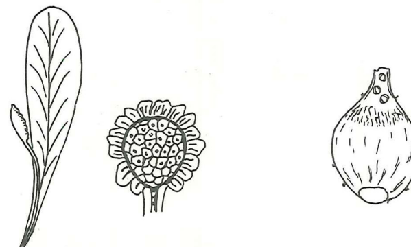
Figur 8. Hunlig reproduktionsorgan på Glossopteris blad. Frøene sidder på den indvendige side af den flade udvækst fra bladets midtnerve. Til højre ses et forstørret frø med pollen i pollen-kammeret (efter J.Schopf og D.Pant).
