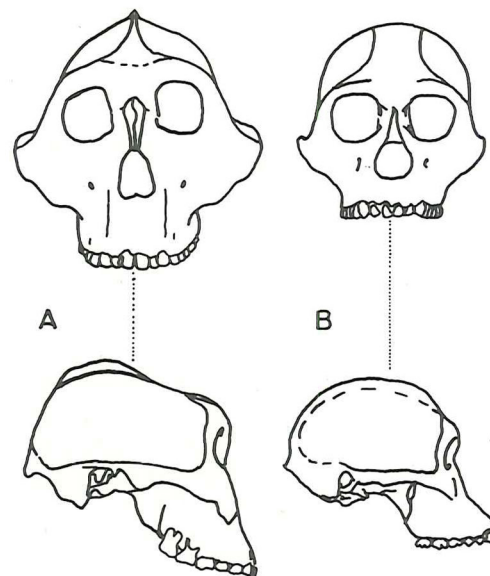
Figur 7. Kranier af australopitheciner set forfra og fra højre. Den robuste form (A) er "nøddesnækker-manden" fra Olduvai, mens den gracile (B) er baseret på fund fra Sydafrika. (Fra Handbuch der Zoologie).
