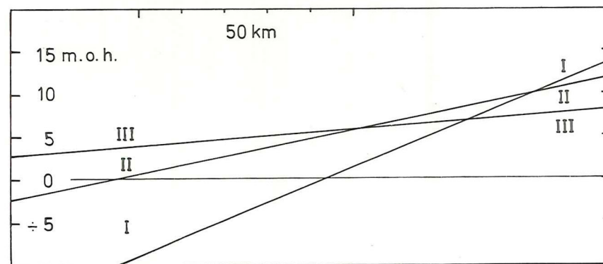
Figur 4. Principskitse af forløbet af postglaciale kystlinier i Nordjylland. (Højderne er kun omtrentlige, I er ældst og III er yngst).
