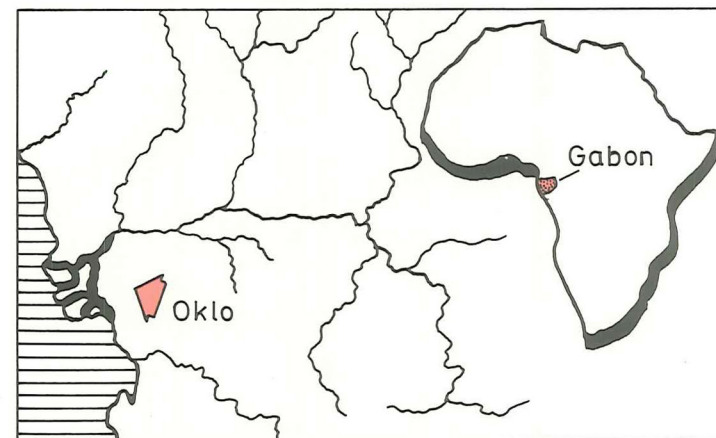
Figur 3. Gabons uran fandtes i tidlig Prækambrium i uranmineraler, der var jævnt fordelt i granit. Efter forvitring af graniten blev uranmineralerne frigjort og skyllet ud i elve. Senere, da atmosfæren blev mere iltholdig, blev uranet iltet til en vandopløselig form. Det opløste uran førtes til deltaområder med organisk materiale, og her blev uranet reduceret til en tungtopløselig form af det organiske materiale, senere er uranet opløst og genafsat i årer og lommer. Se også figur 4 og 5.
