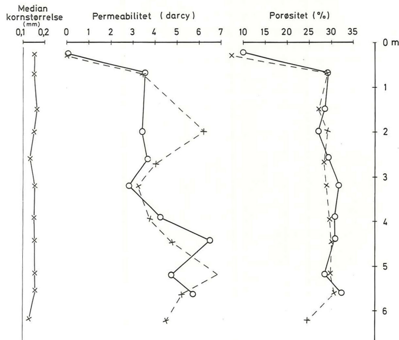
Figur 6. Porositet- og permeabilitetsværdier fra laboratorieundersøgelse af sandstenskerne fra Gassum Formationen. Darcy er en måleenhed for permeabilitet baseret på hastigheden af passage af 1 \text{ cm}^3 vand ved 1 atmosfæres tryk gennem et porøst medium med tværsnitsarealet 1 \text{ cm}^2 og højde 1 cm. Toppen er kalkspatcementeret, hvilket tydeligt afspejles i de målte værdier. Vertikal porøsitet og permeabilitet er markeret med cirkler, horisontal med stjerner (efter Holm & Priisholm 1978).
