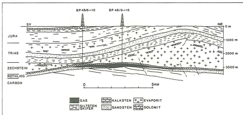
Figur 5. West Sole gasfeltet i den sydlige del af den britiske Nordsø-sektor. Reservoiret ligger i Rotliegendes sandsten under en pudestruktur af Zechstein salt.
