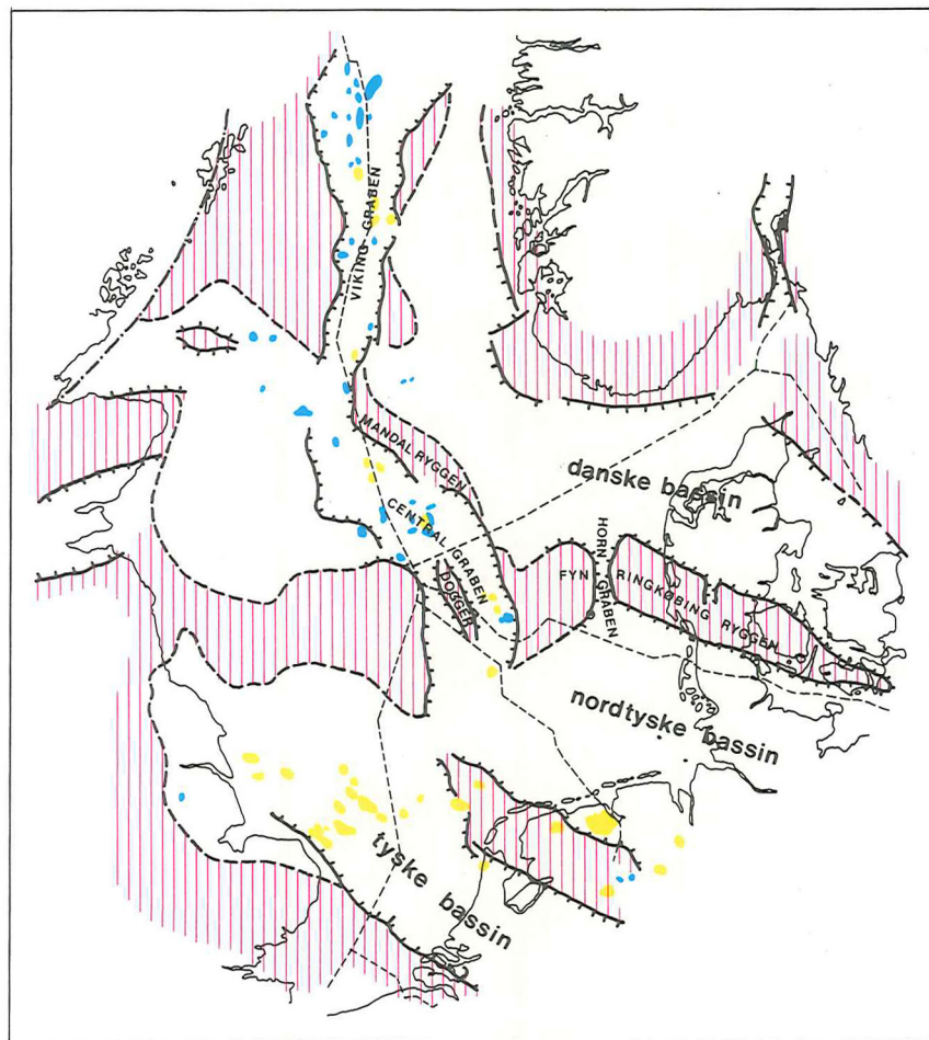
Figur 3. Nordsøens hovedstrukturer. De lodret skraverede områder angiver højtliggende "economic basement" og de takkede linier er betydende forkastningszoner. Blåt er olie-felter mens gult er gas-felter. De stiplede linier er nationale sektorgrænser.
