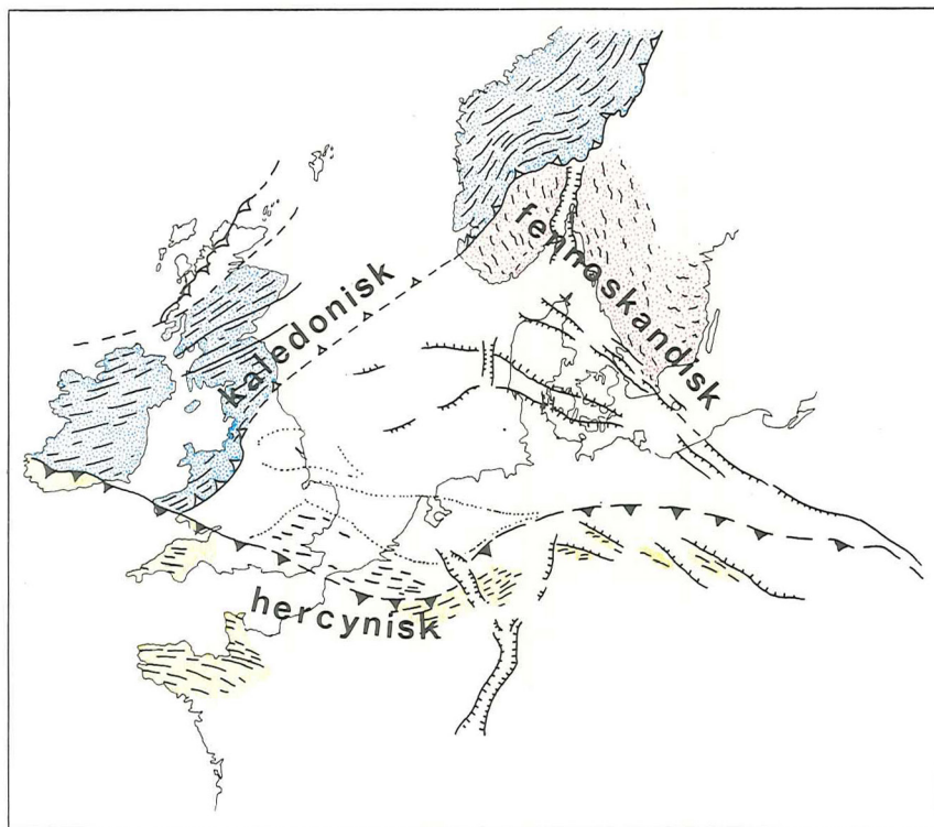
Figur 1. De geologiske hovedstrukturer i Nordeuropa. Nordsø-bassinets område begrænses af henholdsvis den kaledoniske, den variskiske eller hercyniske foldekæde samt det fennoskandiske grundfjeldsskjold.
