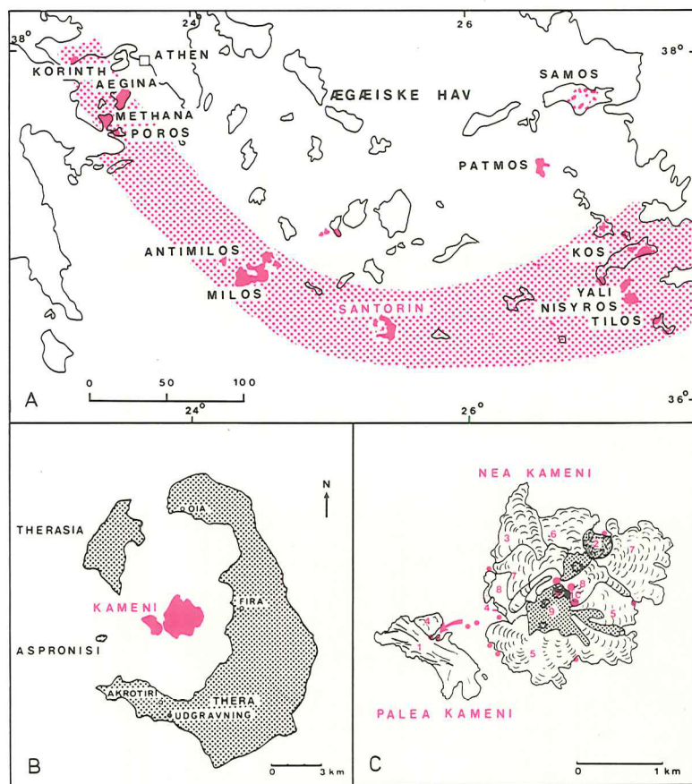
Figur 1. A: Beliggenheden af Santorin og Kyklade øbuen. Yngre vulkanområder er gengivet i rødt. B: Santorin vulkankomplekset med ringøerne Thera, Therasia og Aspronisi, som er næsten fuldstændig dækkede af pimpstenslag fra det sen-minoiske udbrud omkring 1500 f. Kr. De nyere Kameni øer (røde) ligger midt i kalderaen. C: Detailkort over Kameni øerne. Tallene angiver den tidsmæssige rækkefølge af de enkelte lavastrømme, der hidrører fra hver sit udbrud. De større røde cirkler viser, hvor der nu finder gasudstrømning sted (fumaroler). De mindre røde cirkler betegner områder med underøisk jernudfældning. Pilen peger ind i jernbugten.
