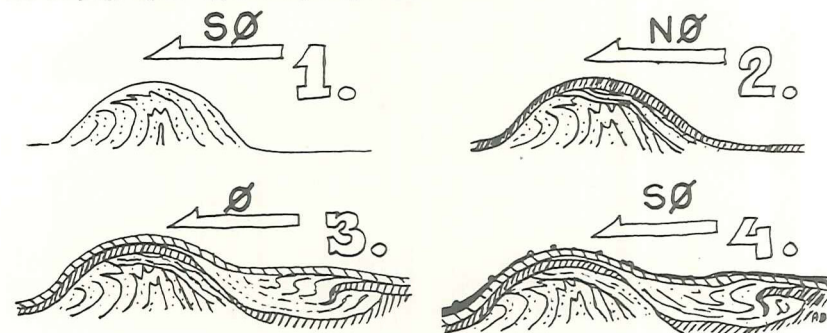
Figur 5. Fire trin i Præstebjergs udviklingshistorie. Pilene angiver hvorfra de forskellige isfremstød kom. Skråskravering er signatur for moræneler.
