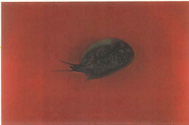
Figur 3. Den marine bladfod Branchiocraris fra den Mellem Kambriske Burgess-skifer (Canada): øverst en skitse, og i midten et parti af bagkroppen. Nederst ses en nulevende bladfod, Lepidocaris, fanget i en københavnsk dam.
