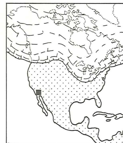
Figur 5. Store dele af Nordamerika var isfrie i Kvartærtiden, og Rancho la Brea området lå langt syd for isranden.
