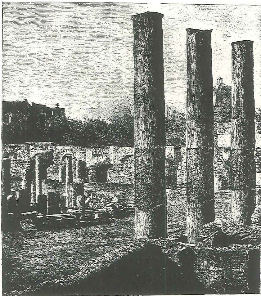
Figur 1. Serapis-templet i Pozzuoli nær Napoli. Den midterste del af søjlerne er angrebet af marine boremuslinger! Efter Nathorst.
