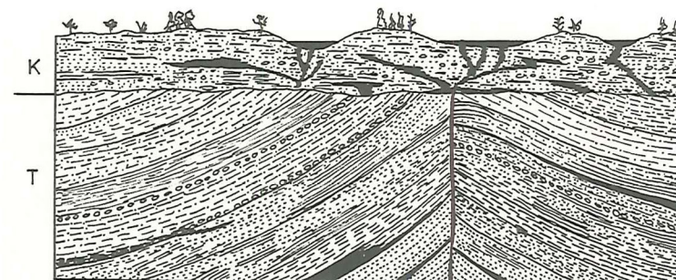
Figur 4. Skematisk snit gennem jordlagene ved Rancho la Brea. I de foldede og forkastede sand- og gruslag fra Tertiærtid (T) er mere porøse lag mættet med olie. I Kvartærtid (K) på godt 50 m er de tidligere oliepøle ved afgasning og tab af mere flygtige kulbrinter blevet til hård asfalt. Flydende asfalt ses som pøle og søer i den nuværende landoverflade. Modificeret efter Arnold.
