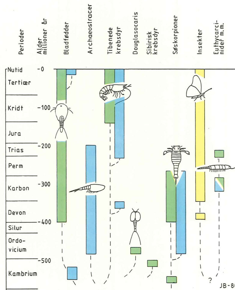
Figur 1. Den kendte geologiske udbredelse af nogle udvalgte leddyrgrupper. Blå farve viser forekomst i havet, grøn farve forekomst i ferskvand og gul farve liv på land. En levevis i ferskvand eller på land, hvor mulighederne for fossilbevarelse er temmelig ringe, kan let give store huller i den tidsmæssige udbredelse.
