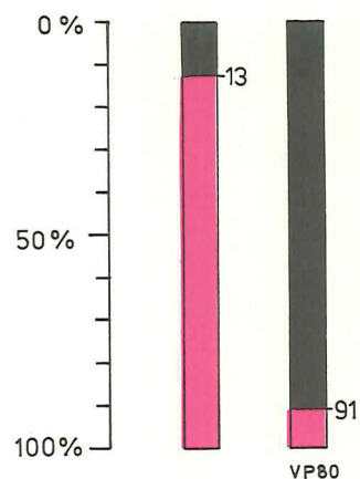
Figur 6. Forholdet mellem rovdyr (sort) og planteædere (rødt) i amerikanske pattedyrfaunaer fra Kvartærtiden. Søjlen til venstre er et gennemsnit af to faunaer fra Oregon og Texas. Søjlen til højre er Rancho la Brea faunaen. Den venstre søjle svarer nogenlunde til fordelingen i en normal nutidsfauna. Data fra Shotwell.
