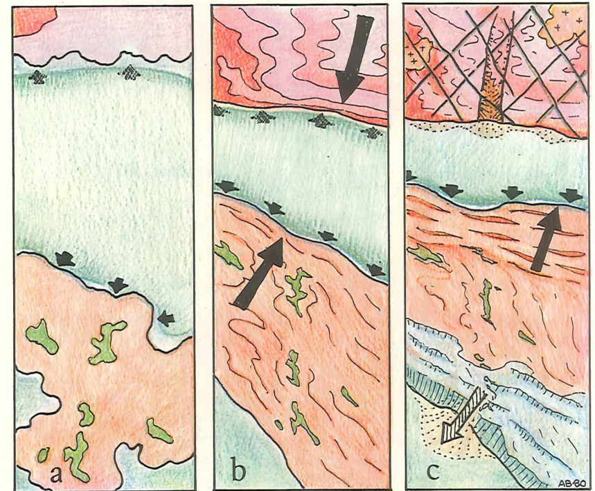
Figur 5. Diagram visende udviklingen i den ældste del af det Baltiske Skjold. Murmansk-kontinentet i nord (øverst) adskilles af Kola-oceanet fra Laplandskontinentet (nederst). a: Situationen for ca. 2,7 milliard år siden, hvor Murmansk-kontinentet er delvis havdækket, og hvor Laplandskontinentet er under dannelse. b: Situationen omkring 2,5 milliard år før nu, hvor pladebevægelser har nærmet de to kontinenter mod hinanden og har medført bjergkædefoldninger. c: Situationen for ca. 2,1 milliard år siden: Laplandskontinentet driver mod nord, dets nordrand foldes, og dets sydrand strækkes.
