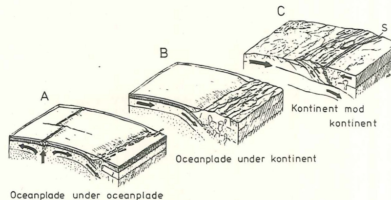
Figur 2. Diagram visende forskellige typer ung pladetektonik. a: ved oceanbundsspredning omkring midt-oceanisk ryg tvinges oceanplade ned under oceanplade, og en dybgrav og en øbue opstår. b: Oceanpladen tvinges ned under randen af en kontinentplade, - eksempel Andesbjergene. c: Oceanet lukkes, så kontinenterne i to modgående plader bringes til kollision. Rester af den gamle oceanbund (S) angiver den oprindelige pladegrænse, - eksempel Himalaya.
