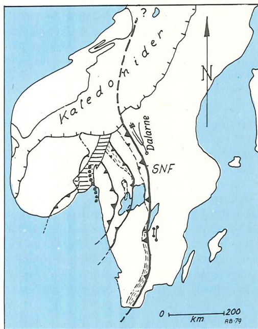
Figur 1. Skitse af Sydskandinavien visende de vigtigste forskydningszoner i det Svekonorvegiske foldestrøg. SNF står for den Svekonorvegiske front mod ældre grundfjeld i Syd- og Mellemsverige. Det Permiske Oslo-felt er vandret skraveret.
