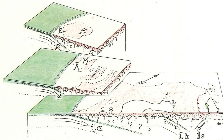
Figur 3. Blokdiagram visende tre stadier i det Baltiske skjolds vækst. Den forreste blok viser situationen for ca. 1750 millioner år siden under den Svekofeniske foldning. I a, b og c er formodede subduktionszoner. Den mellemste blok viser udviklingen omkring 1650 millioner år før nu - efter anlægget af en ny subduktionszone, der medførte at endnu et bælte oceanisk skorpe blev omdannet til kontinent-skorpe. Det bagerste diagram viser situationen for ca. 1500 millioner år siden, hvor endnu en ny jordskorpe-bræmme på samme måde var blevet føjet til skjoldet. Det mellemste og bagerste diagram viser udviklingsstadier, der senere blev ændret under den Svekonorvegiske foldning, som medførte kraftig jordskorpe-forkortelse. E: Egersund, A: Arendal, M: Moss, S: Stockholm, L:Luleå. Oceanisk skorpe er grøn, kontinent-skorpe rød.
