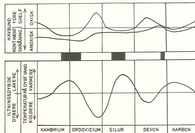
Figur 5. Skematisk fremstilling af faktorer førende til udbredelse af sortskifer. Kurverne angiver kun relative tendenser i forhold til de vandrette linier, der kan repræsentere en tænkt middeltilstand. Sorte felter viser større udbredelse af sortskifer. Se teksten angående tolkning. Stærkt modificeret efter Berry & Wilde.
