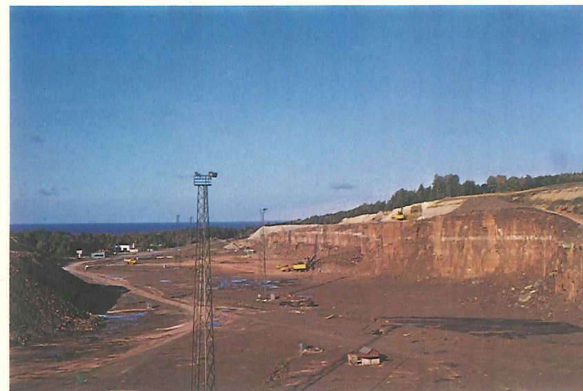
Figur 2. Kalkstensbruddet ved den nu nedlagte fabrik i Hällekis ved Kinnekulle i Västergötland.
