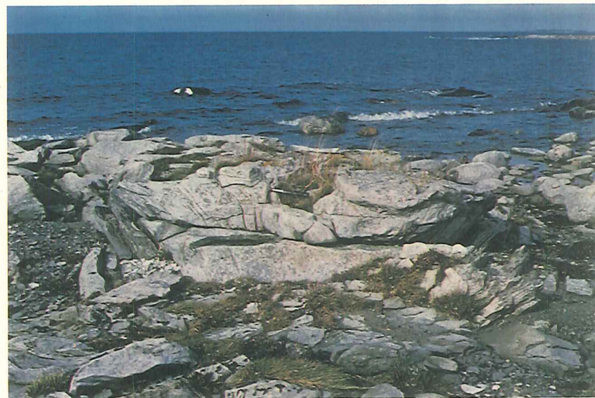
Figur 1. Sedimentfolder i silurisk Burgsviksanden fra Kulhaken på Sydgotland. Foto Sven Laufeld.
