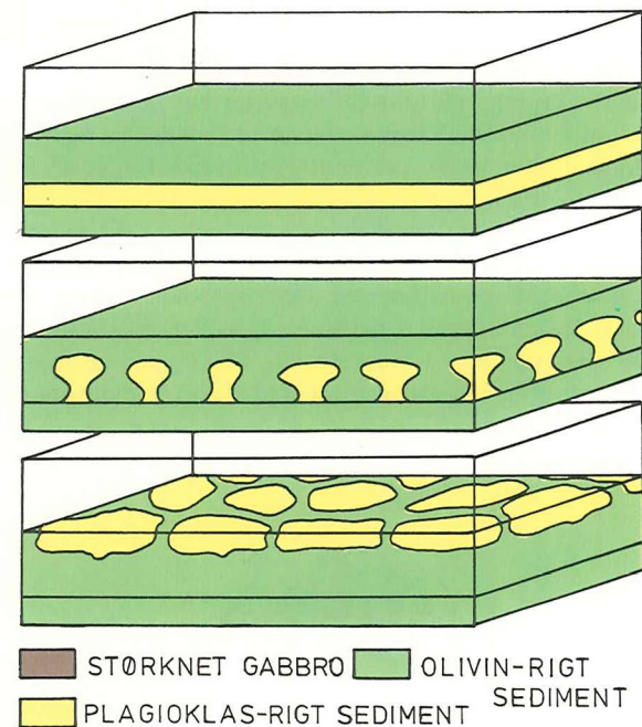
Figur 6. Skematisk tolkning af strukturerne i figurerne 4 og 5. Fremadskridende deformation fra A til C. Stadium A umiddelbart før deformationen starter, stadium B svarer til fig. 4, stadium C svarer til fig. 5. Næste stadium ville ikke kunne adskilles fra en eventuelt primær, stabil fordeling (plagioklas på toppen af olivin-rigt lag).
