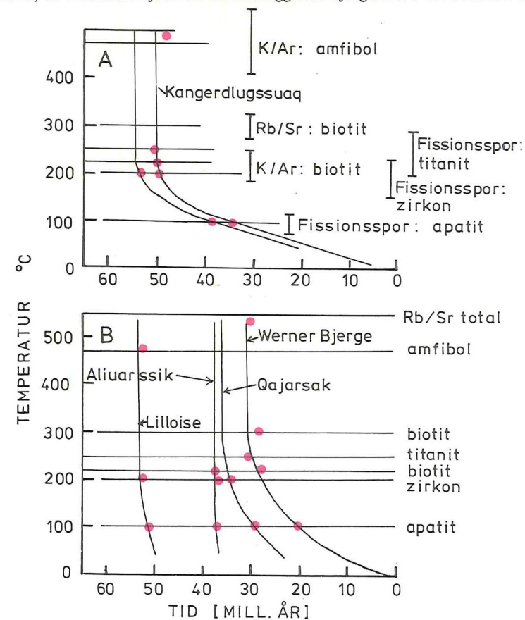
Figur 3. Diagrammer visende afkølingsforløbet for de daterede terciære intrusioner. Øverst (A) intrusioner fra domens centrale del, nederst (B) fra domens ydre del. Efter Brooks og Gleadow (1979). Tid i millioner år.
