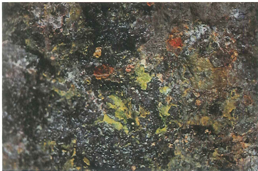
Figur 3. Wölsendorfit (orange) og beta-uranofan (gult) i biotit-pegmatit fra Luleå Manak, Lapland. Foto Runo Löfvendahl.
