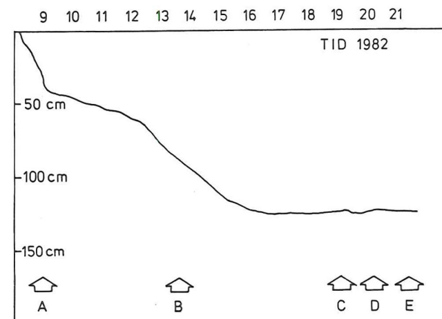
Figur 3. Sætningsforløbet igennem hele fasen fra skreddets start til vejens retablering. Talrækken øverst viser ugenumre. A: Afgravning påbegyndt. B: Skinneramning påbegyndt. C: Skinneramning afsluttet. D og E: Færdigetablering af vej og opfyldning.
