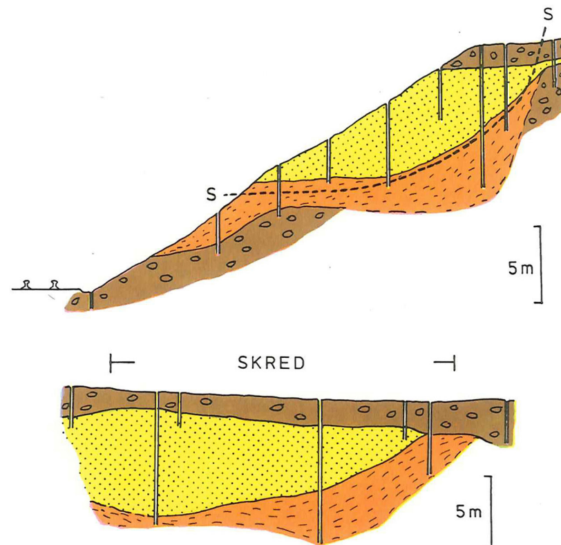
Figur 6. Boreprofiler gennem skredområdet. Øverst ses et tværsnit igennem skreddet. Skredfladen er vist med stiptet linie. Lodrette streger angiver borer. Med brun farve er vist moræner, lilla farve angiver "brokkeler", og rød farve viser finkornet, ensartet smeltevandssand. Nederst et profil igennem skreddet langs med banen i vejsiden. Samme farver som øverst.
