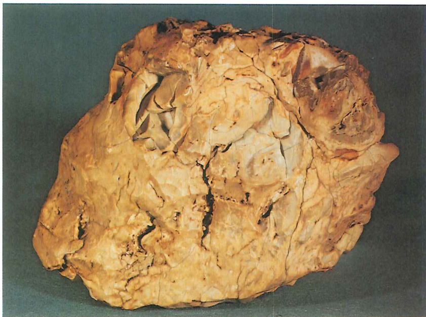
Figur 2. Breccieret flintkonglomerat fra Vestjylland. Foruden enkelte afrundede flintstykker ses breccierede partier, der er svære at skelne fra den finkornede grundmasse. Foto: Ole Bang Berthelsen.
