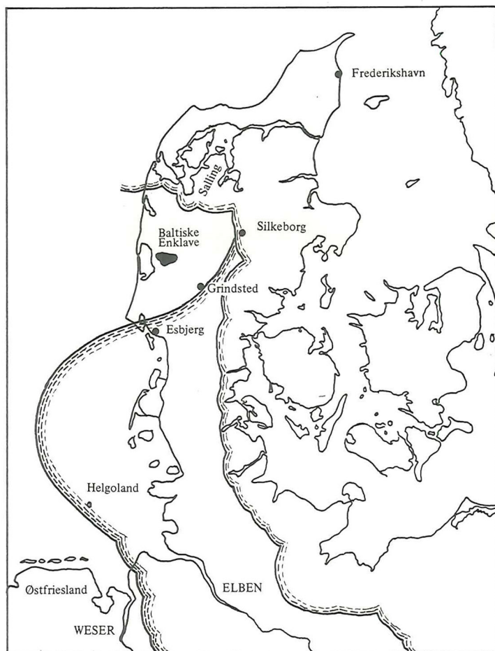
Figur 9. Kort over den formodede udbredelse af det sene Saale (Warthe) isfremstød tværs over det sydlige Jylland og Nordtyskland frem til Esbjerg-Grindsted-Silkeborg-linien i nordvest og fra Helgoland til Weser floden i sydvest. Endvidere er israndslinien for det maksimale isfremstød i Weichsel indtegnet i det centrale Jylland (Hovedopholdslinien).
