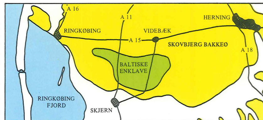
Figur 8. Området omkring den Baltiske Enklave. Bakkeøer er vist med gult, enklaven med grønt. Landområder uden farve er yngre end Saale-istiden.
