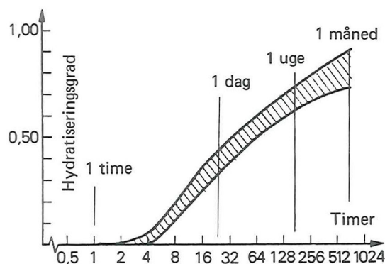
Figur 1. Dannelsen af betonens bindemiddel, cementpastaen, sker ikke i løbet af en enkelt nat. Hydratiseringen af klinkerkomponenterne foregår over længere tid, og selv efter 1 måned er kun godt 80 % af cementpastaen blevet færdigdannet.
