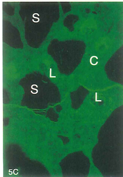
Figur 5. Tyndslipsbilleder af revnet beton. A: set i almindeligt gennemfaldende lys. En revne ses på grund af limens indhold af gult farvestof. Tæt ved revnen ses en farveændring i pastaen, der her indeholder mere farvestof. I to luftporer ses radiært stillede nåleformede krystaller. B: samme udsnit set i polariseret lys med gipsblad i strålegangen. Der ses en forskel i formen på CH-kornene i den smalle omdannede zone om revnen sammenlignet med den uomdannede pasta. De radiært stillede krystaller kan identificeres som Aft-fase. C: Samme udsnit set i fluorescerende lys. Ændringen i porøsiteten af den omdannede pasta træder nu tydeligere frem. S=sand, C=cementpasta og L=luftporer. Format: 1.08x0.75 mm.
