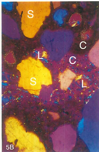
Figur 5. Tyndslipsbilleder af revnet beton. A: set i almindeligt gennemfaldende lys. En revne ses på grund af limens indhold af gult farvestof. Tæt ved revnen ses en farveændring i pastaen, der her indeholder mere farvestof. I to luftporer ses radiært stillede nåleformede krystaller. B: samme udsnit set i polariseret lys med gipsblad i strålegangen. Der ses en forskel i formen på CH-kornene i den smalle omdannede zone om revnen sammenlignet med den uomdannede pasta. De radiært stillede krystaller kan identificeres som Aft-fase. C: Samme udsnit set i fluorescerende lys. Ændringen i porøsiteten af den omdannede pasta træder nu tydeligere frem. S=sand, C=cementpasta og L=luftporer. Format: 1.08x0.75 mm.
