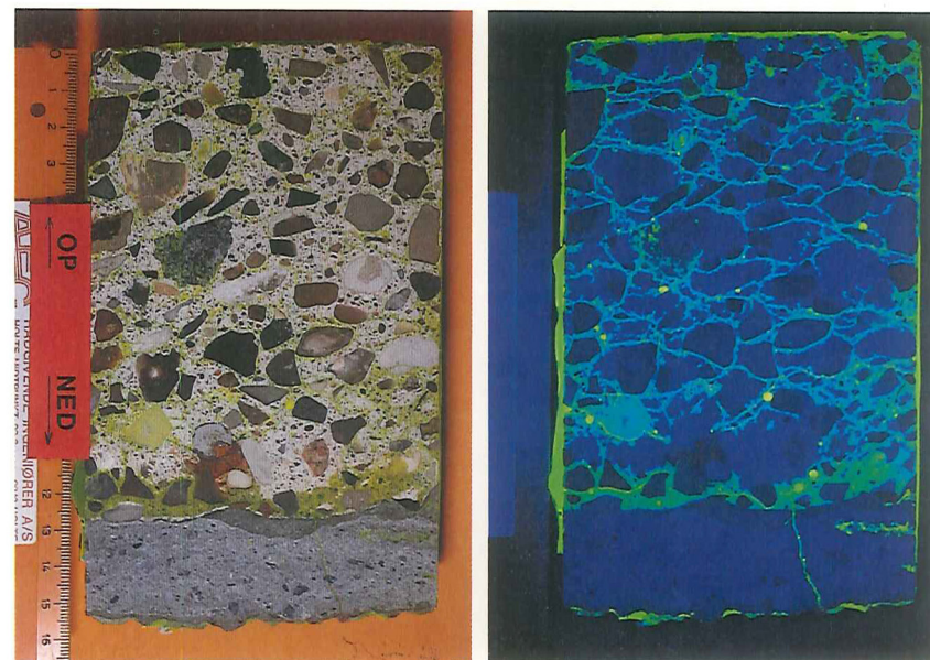
Figur 4. Planslib af borekerne af beton fremstilles ved at save kernen igennem i midterplanet og polere skæreflader. Herefter imprægneres fladen med et farvestof. Til venstre ses kernen i almindeligt lys, til højre i ultraviolet lys, hvor farvestoffet får revnebilledet til at træde tydeligt frem.
