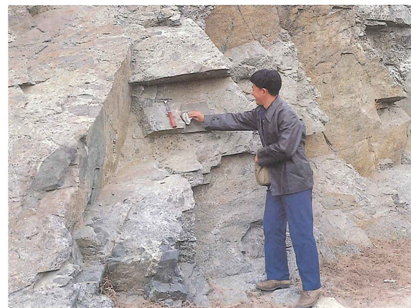
Figur 9. Amfibolit facies gnejser fra den nordlige del af Hebei provinsen. Europæiske geologer kortlagde bjergarten som en granitisk gnejs med indeslutninger af mørkt materiale. Kineserne lægger mere vægt på indeslutningerne og ville beskrive enheden som en vulkansk bjergart, der var blevet brudt i stykker af sene Arkæiske granitårer.
