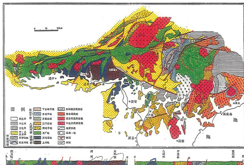
图1 冀东早前寒武地质图
