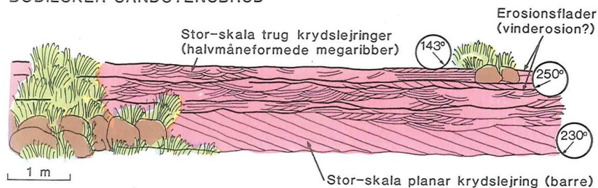
Figur 3. Profilskitse fra det sydøstlige hjørne af Bodilsker Sandstensbrud. De indcirklede tal angiver gennemsnit af strømretningsmålinger for bænke.
