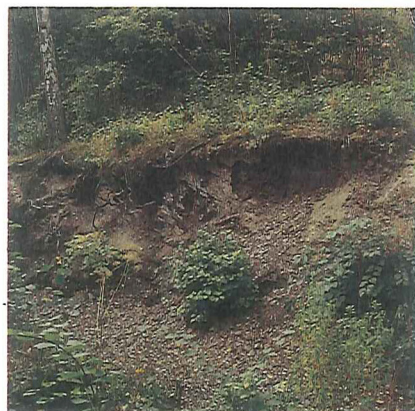
Figur 26. Cyrtoagraptus Skifer i den vestlige brink af Øleå ved lokalitet P-12. Foto: Valdemar Poulsen.
