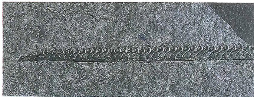
Figur 27. Graptoliter fra Cyrtograptus Skiferen , alle tilhørende slægten Mono-graptus . Øverst er graptoliten bevaret i relief på grund af udfyldning med svovlkis, i midten er den organiske kulhinde væk, så svovlkis udfyldningen er synlig, og nederst er graptoliten fladtrykt, hvilket er det mest almindelige. Foto: Ole Bang Berthelsen og Jan Aagaard.
