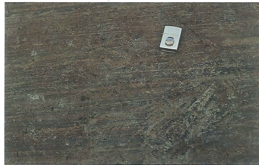
Figur 23. Iस्कuret overflade med tværsnit af en orthoceratit, der er omkranset af slagmærker efter mange forgæves forsøg på at hamre den fri. Indtil for få år siden var stykket pænt bevaret. Foto: Valdemar Poulsen.
