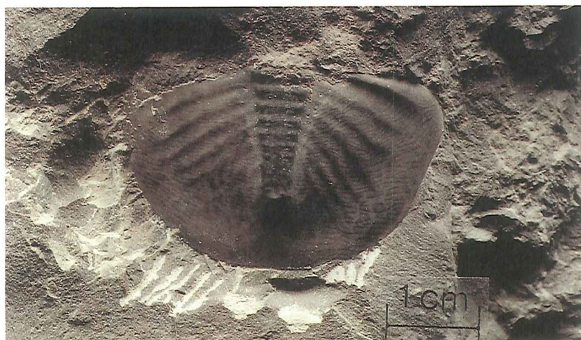
Figur 24. Trilobiter (hale) fra Komstad Kalken ved Skelbro. Øverst er en Megistaspis, og nederst ses en 'Ptychopyge'. Foto: Jan Aagaard.
