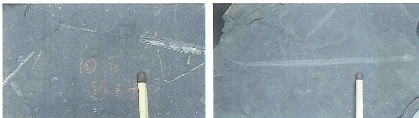
Figur 17. Graptoliter fra Dicellograptus Skiferen. Til venstre Dicellograptus (V-formet) og Orthograptus . Til højre ses 'Diplograptus' (nederst) og 'Climacograptus' (øverst). Foto: Ole Bang Berthelsen.
