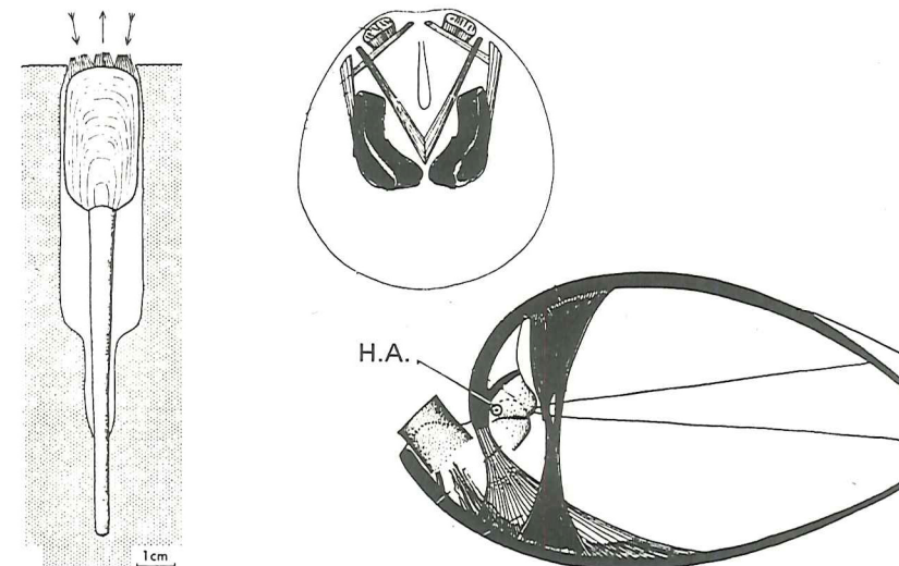
Figur 1. Til venstre ses Lingula i livsstilling. Øverst til højre ses musklerne hos den hængsellose Crania. Dorsalskallen er fjernet. Nederst til højre er der et længdesnit af Terebratulida. H.A. er hængselaksen, sort er lukkemuskler og stribet er åbnemuskler, skræmmuskler og stilkfasthæftningsmuskler. Hos de hængsellose brachiopoder bruges skræmmusklerne til at rotere skallerne i forhold til hinanden, så uønsket sediment slynges bort. Hos de hængslede former har stilmusklerne samme funktion, idet dyret kan rotere i små ryk om stilken.
