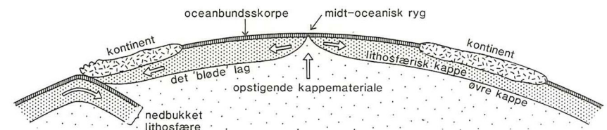
Figur 1. Skematisk snit gennem Jordens yderste lag visende pladernes opbygning og bevægelse. Ny oceanbundsskorpe dannes til stadighed langs den midt-oceaniske ryg, hvor pladerne glider fra hinanden på 'det bløde lag', astenosfæren. 'Pladeproblemet' løses ved, at oceanbundsskorpe med vedhængende stive kappe (lithosfæren) andre steder bukket ned og genoptages i den dybere kappe.
