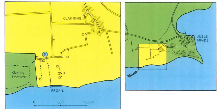
Figur 1. Klinten, som omtales i denne artikel, ligger ca. 800 meter øst for Albæk Hoved på nordsiden af Vejle Fjord. Er man kørende i en ikke for stor bil, kan man parkere i vejsiden som vist på kortet. En privat markvej fører herfra ned til den vestlige ende af klinten. Man skal indhente tilladelse til at færdes på markvejen hos planteskoleejer Bent Sørensen, Stationsvej 37, Klaking, 7130 Juelsminde (tlf.: 75 69 31 34). Ellers må man fortsætte til fods gennem Klaking Skovhaver og nå kysten vest for profilet.
