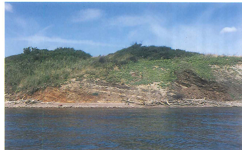
Figur 15. Overgangen mellem Røsnæs Ler og Lillebælt Ler på strækningen fra 150 til 190 meter. Det grå lag med to næsten hvide mergelbænke er lag R6. Det brune ler til højre er lag L1 i Lillebælt Leret.
