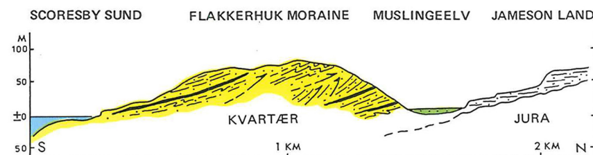
Figur 3. Skematisk snit gennem Flakkerhuk morænen. De tykke sorte lag er moræner (till). I øvrigt opbygges ryggen af tidevandsprægede marine sedimenter.
