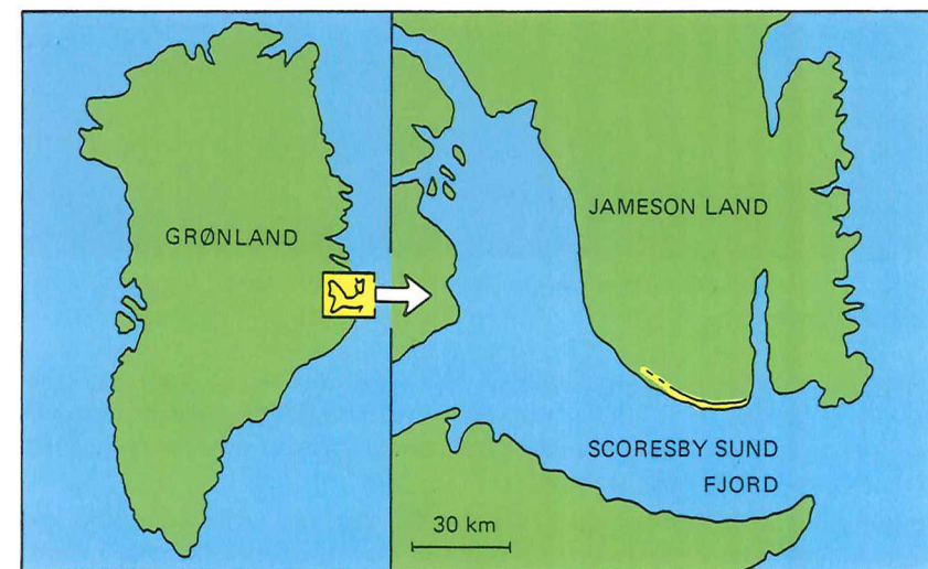
Figur 1. Det undersøgte område i Østgrønland. Flakkerhuk morænen, der er vist med gult, ligger på det sydlige Jameson Land.
