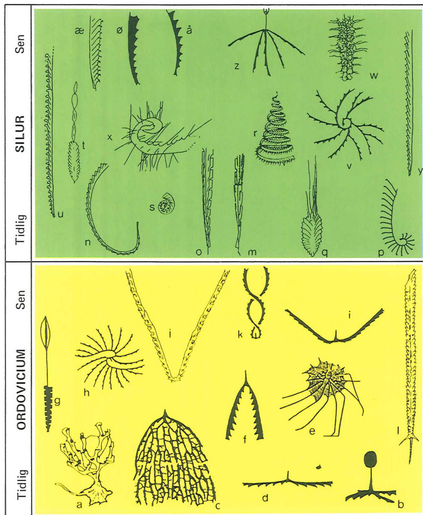
Figur 4. Diagram som viser graptoliternes mangeartede koloniformer gennem Ordovicium og Silur. a: Dictyonema (fastsiddende form), b–å: fritlevende former. b: 'Staurograptus', c: Rhabdinopora, d: Didymograptus, e: Loganograptus, f: Didymograptus, g: Pseudoclimacograptus, h: Nemagraptus, i: Leptograptus, j–k: Dicellograptus, l: Orthograptus, m: Akidograptus, n: Coronograptus, o: Rhaphidograptus, q og t: Petalograptus, r, s, u, x, ø og å: Monograptus, z: Linograptus. (Efter Bates & Kirk, Bulman og Müller).
