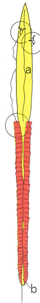
Figur 11. Rekonstruktion af graptoliter Cystograptus vesiculosus . I de to øverste cirkler ses individer, med eller uden stilk, som man har forestillet sig kunne bevæge sig ud af thekerne for at konstruere de store membraner (a). Bemærk den relativt lange vej, de små individer må have bevæget sig. Orange farve er theker. Nederst (b) ses sicula.
