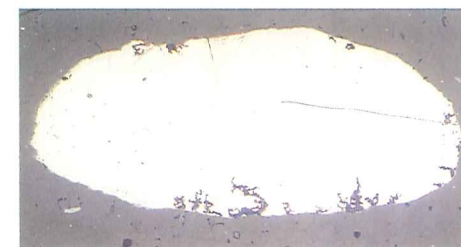
Figur 4. Afrundet stålfragment i den glasagtige bjergart. Kornet er 2.5 mm langt. Poleret prøve set i reflekteret lys. Herunder del af samme korn, nu med ætset overflade, som viser mikrostrukturer, der tillader bestemmelse af kornets opvarmnings- og afkølingshistorie.
