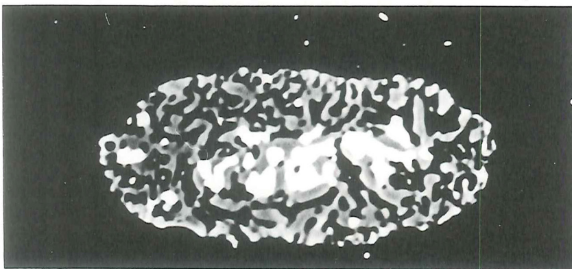
Figur 3. Et reflekteret elektronbillede af et oprindelig jern-titan-oxidkorn, der er rekrystalliseret til rutil (grå) og jernsulfid (hvid). Langs kornets yderste rand ses det nydannede mineral armalcolit. Kornet er ca. 0.04 mm langt.
