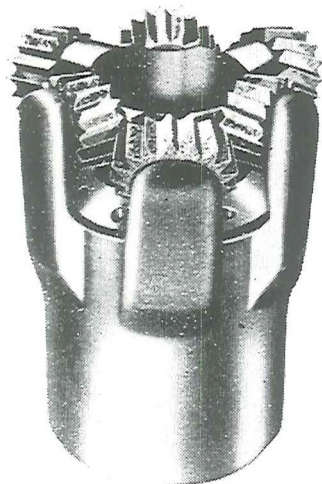
Figur 5. Borekrone med rullemejsler.
