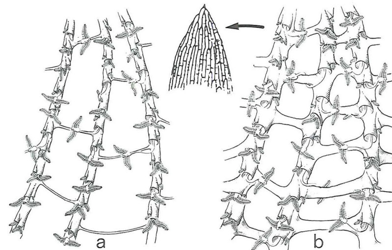
Figur 3. Skematisk rekonstruktion af en del af a: et ungt eksemplar og b: et fuldt udvokset eksemplar af Rhabdinopora flabelliformis. Det udvoksede eksemplar har tykkere grene på grund af et mere veludviklet cortikallag, som tænkes dannet af de individer, der er kravlet ud af thekerne (efter Erdtmann).
