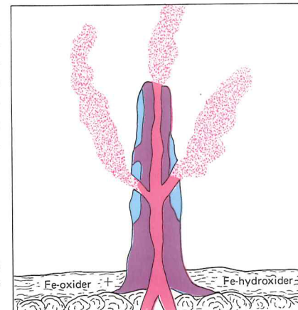
Figur 4. Opbygningen af en black smoker. Varme fluid er rosa, sulfider er violette og sulfater blå.
