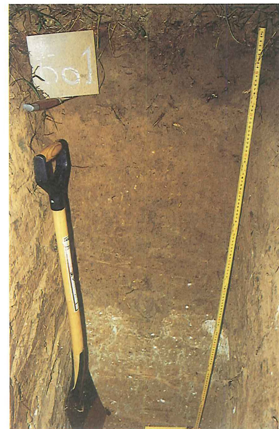
Figur 3. Brunjordsprofil i kalkholdig moræner fra Sjælland. Foto: Leif Petersen.
