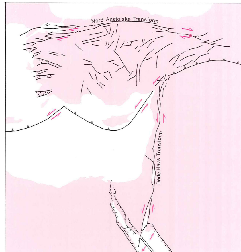
Figur 3. Forkastningsmønstret i Tyrkiet. Linier med korte sidestreges angiver lokal strækning, medens linier med trekantner angiver subduktions-zoner. Øvrige linier angiver sideværts forkastning. Placeringen af byen Erzurum er vist med en rød plet.
