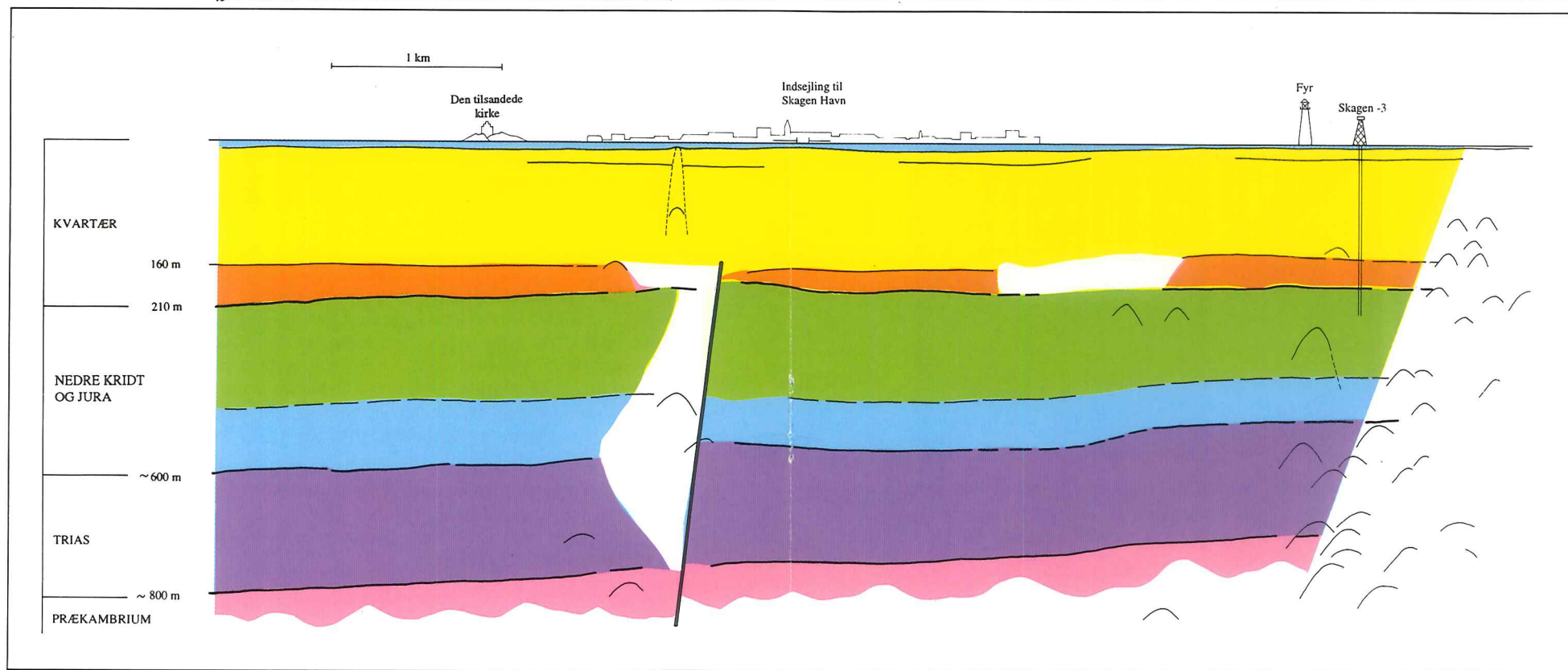
Figur 2b. Fortolkning af det seismiske profil vist i fig. 2a.
