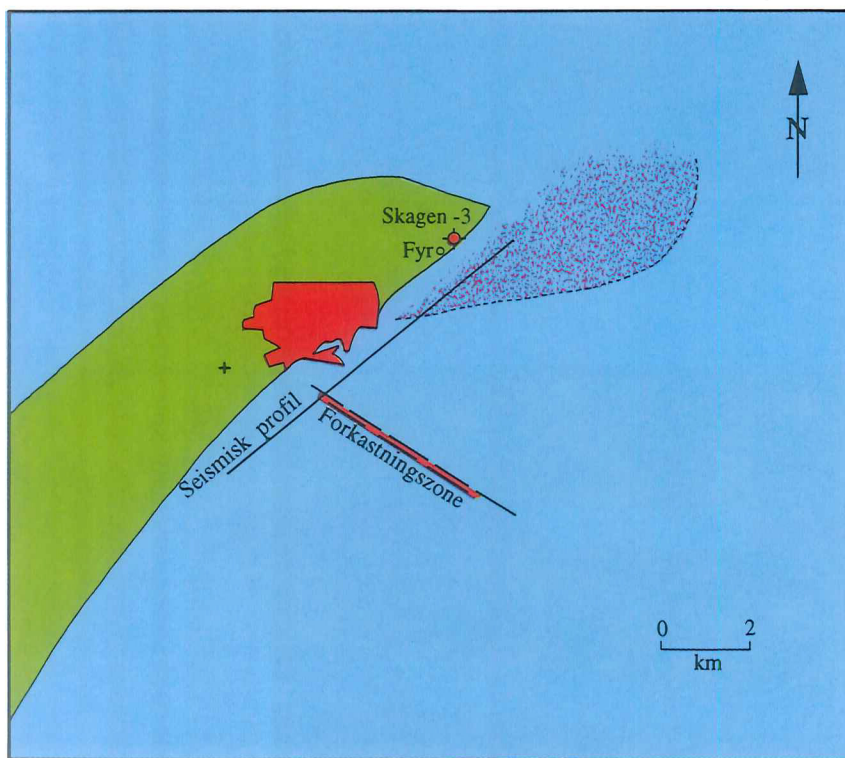
Figur 3. Kort over udbredelsen af gas i overfladenære aflejringer nordøst for Skagen (violet raster). Forløbet af den formodede forkastningszone er vist ligesom beliggenheden af det seismiske profil i fig. 2. Krydset sydvest for Skagen angiver placeringen af den tilsandede kirke.
