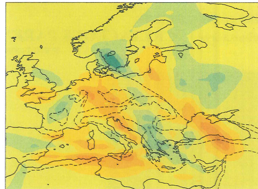
Figur 7. Tomografi fra 300 km's dybde optaget af A. Zielhuis 1993
