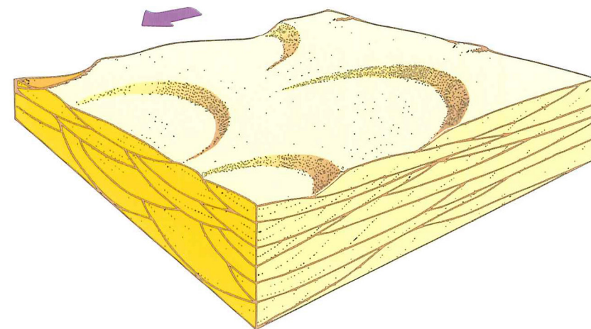
Figur 5. Skematisk model for dannelse af trugkrydslejrning. Den karakteristiske konkave undergrænse dannes ved erosion i truet foran de migrerende megaribber. De skrå forsæt dannes ved episodisk nedskridning af materialet på megaribbens stejle læside. Ved nedskridningen sker en sortering af materialet, hvilket gør hvert enkelt nedskrid synligt. De aflejringer, som dannes af den enkelte megaribbe, bliver udsat for erosion af den efterfølgende megaribbe. Hvis der er tilstrækkeligt materiale til rådighed, eller hvis strømhastigheden aftager, kan dele af megaribberne blive bevaret som trugkrydslejrning. Ved mangel på materiale eller ved en stigning i strømhastigheden sker erosion, og tidligere dannede trugkrydslejringer kan blive fjernet.
