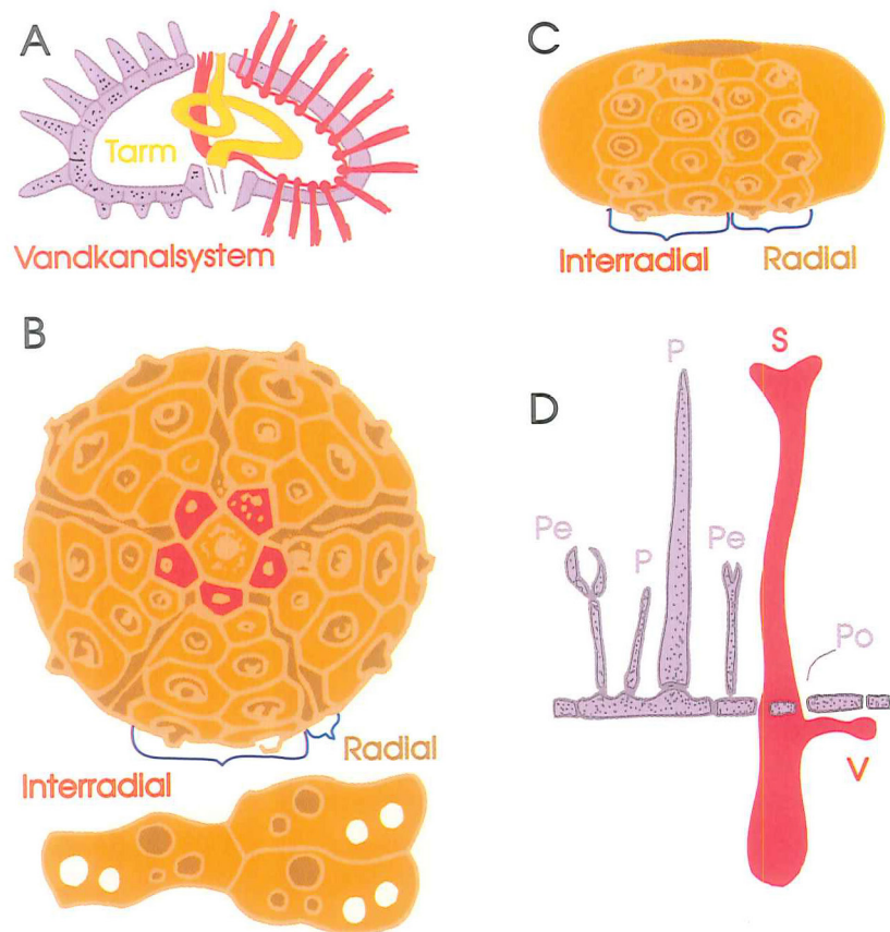
Figur 1. A: Snit gennem et regulært søpindsvin. B: Skallen af griffelsøpindsvin ( Cidaris ). I midten ses topfeltet, hvor gattet er omgivet af 5 store genitalplader, der hver bærer en pore til frigørelse af kønsprodukter. Forneden 3 stærkt forstørrede radialplader. C: Phymosoma -skal fra skrivekridt. Kun et radiale og et interradiale er angivet. D: snit gennem interradiale- og radiale plader. P = pig. Pe = pedicellarie, det er en omdannet pig, der ender i en slags knibtang. De bruges til at rense søpindsvinets overflade. Den største pedicellarie har giftkirtler og kan dræbe f. eks. muslinge- og kalkrørsorms-larver, der vil slå sig ned. Po = porer til podierne. S = sugefod (podie med sugekop på enden). V = radiale vandkanal.
